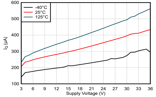
图 5-18. 静态电流与电源电压间的关系
