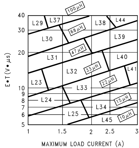
图 7-5. LM2670 — 可调节
