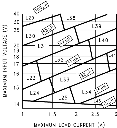
图 7-4. LM2670 — 12V
