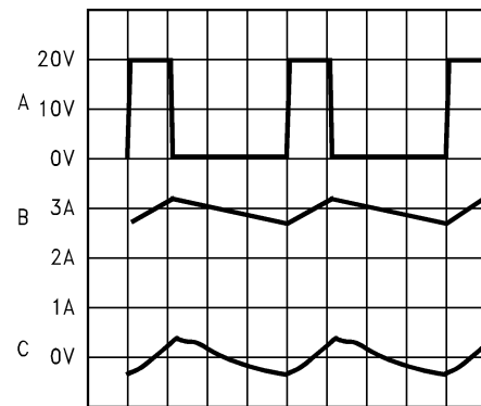
图 5-10. 开关频率
