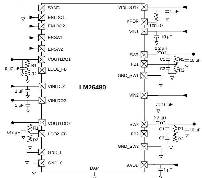
简化原理图
