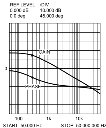
图 7-2. 调制器的增益和相位， R_{\text{LOAD}} = 50\text{hms} 且 C_{\text{OUT}} = 177\mu\text{F}
