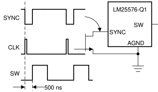
图 6-3. 与外部时钟同步
