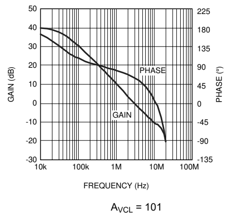
图 5-6. Error Amplifier Gain and Phase
