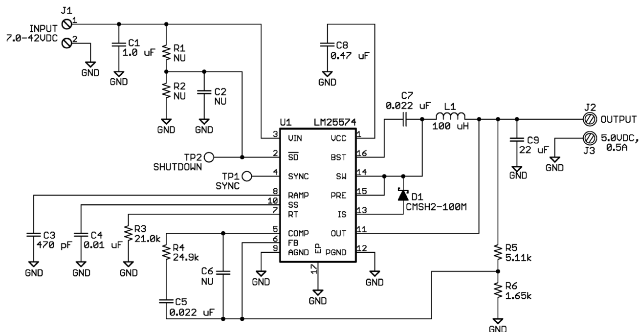
图 7-1. LM25574 Reference Schematic
