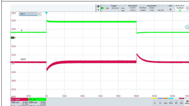
图 7-10. Load Regulation
