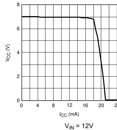
图 5-4. V_{CC} vs I_{CC}
