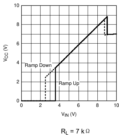
图 5-5. V_{CC} vs V_{IN}
