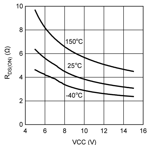
图 5-4. HO High R_{DS(ON)} vs VCC
