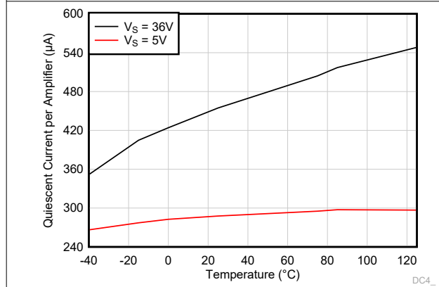
图 5-23. 静态电流与温度间的关系
