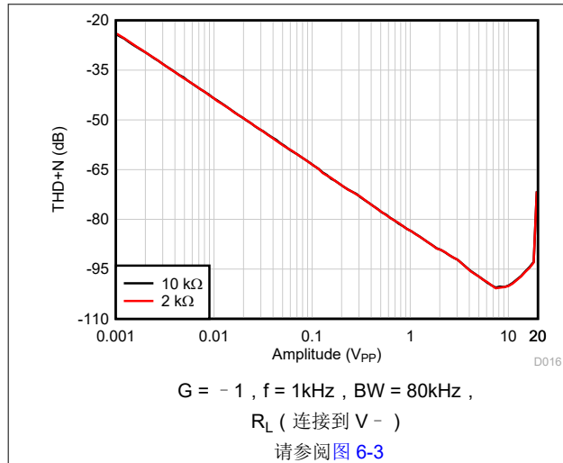
图 5-21. THD+N 比与输出振幅间的关系， G = -1
