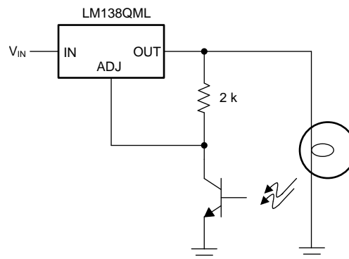
图 31. Light Controller
