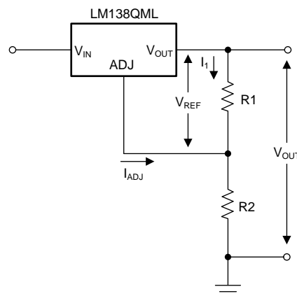
典型应用电路
