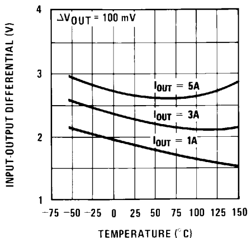
图 5. Dropout Voltage
