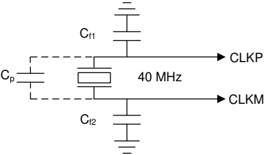
图 7-10. 晶体实现方式
