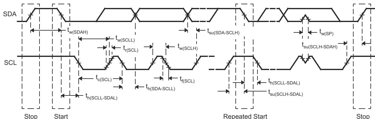
图 7-17. I2C 时序图
