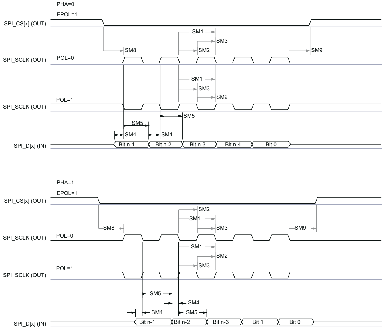
图 7-11. SPI 时序 — 控制器模式接收
