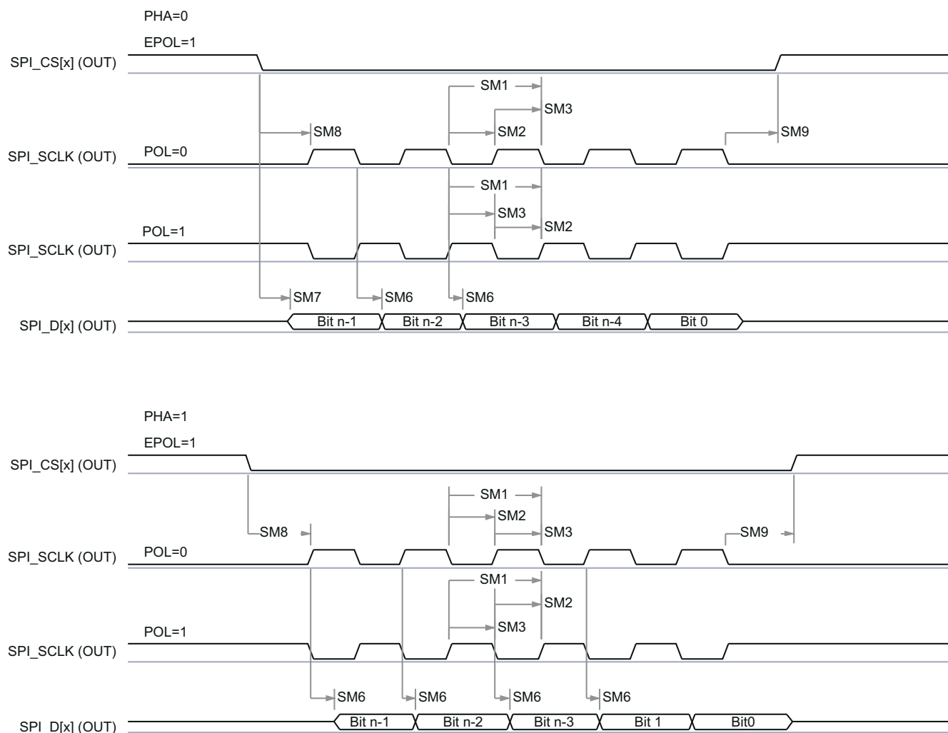
图 7-12. SPI 时序 — 控制器模式发送
