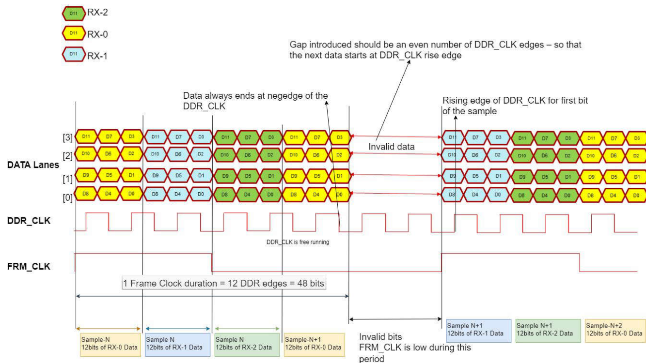
图 7-16. RDIF 数据格式
