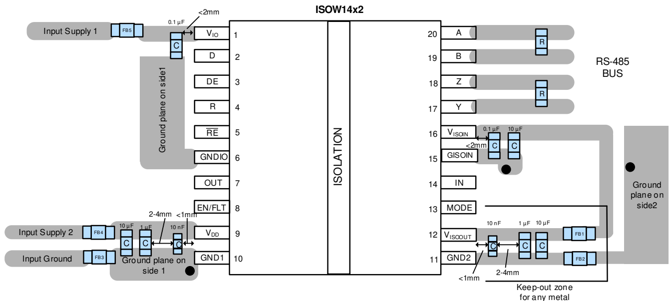
图 13-1. Layout example
