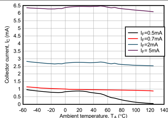
ISOM8110 和 ISOM8115 V_{CE} = 5\text{V}
