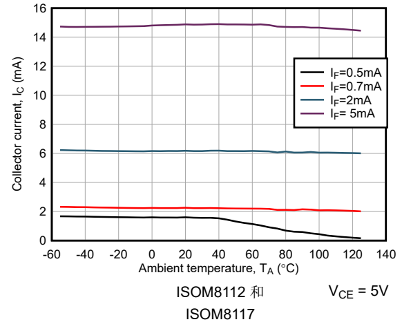
图 6-20. 集电极电流与环境温度间的关系
