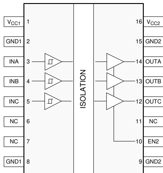
图 4-1. DW 和 DWW 封装 16 引脚 SOIC 顶视图
