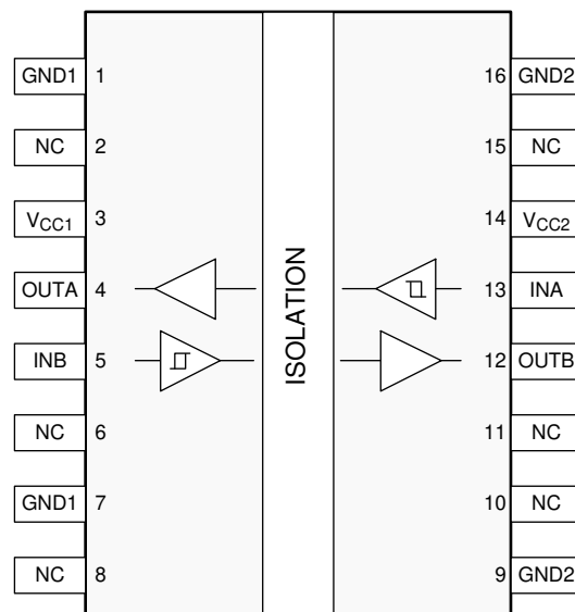
图 5-2. ISO7721-Q1 DW 封装 16 引脚 SOIC 顶视图
