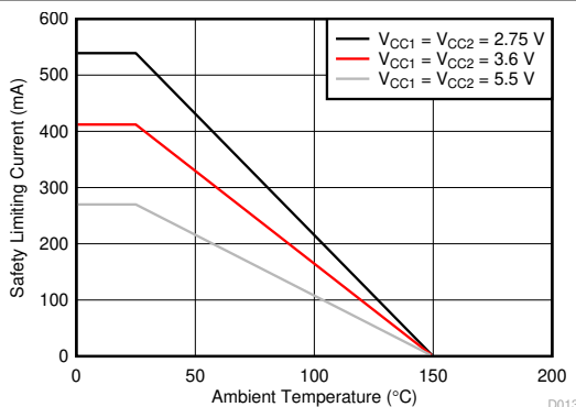
图 6-3. DWV-8 封装根据 VDE 标准限制电流的热降额曲线
