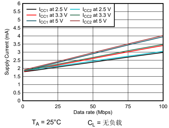
图 6-10. ISO7721-Q1 电源电流与数据速率间的关系 (无负载)
