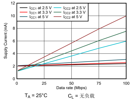
图 6-8. ISO7720-Q1 电源电流与数据速率间的关系 (无负载)
