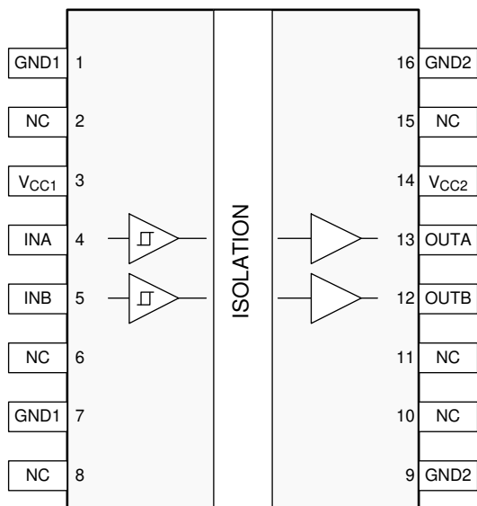
图 5-1. ISO7720-Q1 DW 封装 16 引脚 SOIC 顶视图
