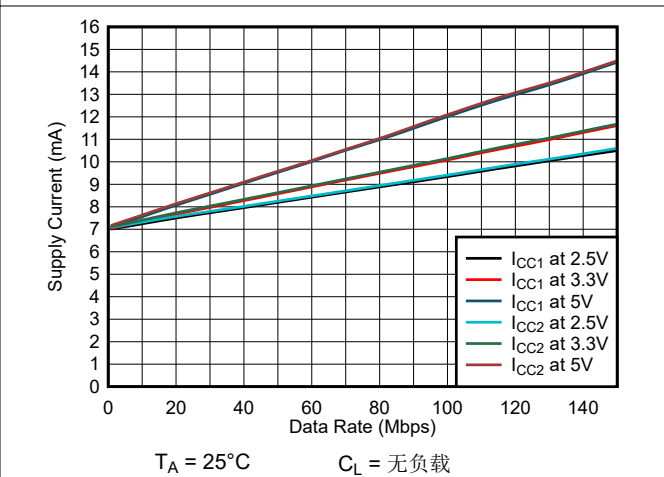
图 6-6. ISO6463 或 ISO6463F 电源电流与数据速率间的关系 (无负载)
