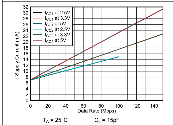
图 6-5. ISO6463 或 ISO6463F 电源电流与数据速率间的关系 (15pF 负载)
