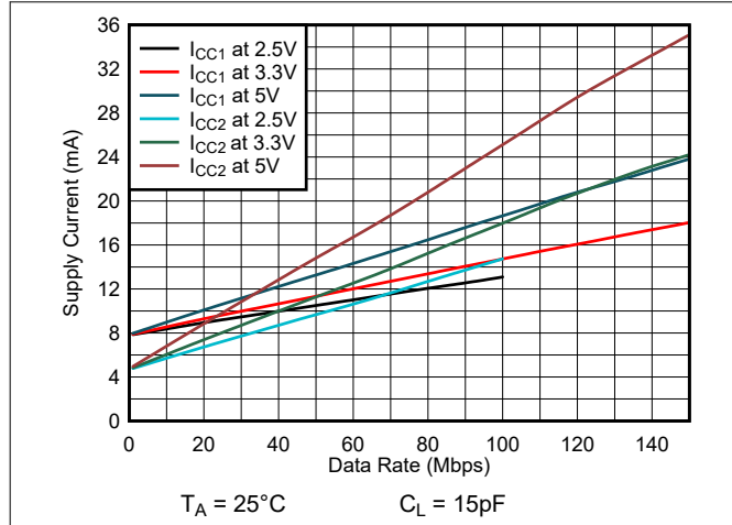
图 6-3. ISO6462 或 ISO6462F 电源电流与数据速率间的关系 (15pF 负载)
