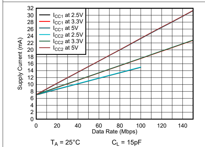
图 6-5. ISO6463 或 ISO6463F 电源电流与数据速率间的关系 (15pF 负载)
