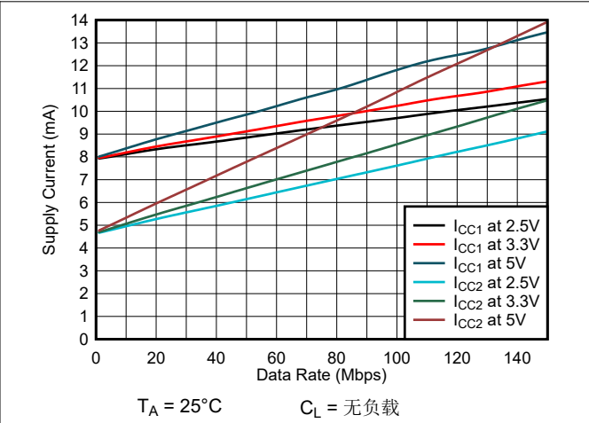
图 6-4. ISO6462 或 ISO6462F 电源电流与数据速率间的关系 (无负载)
