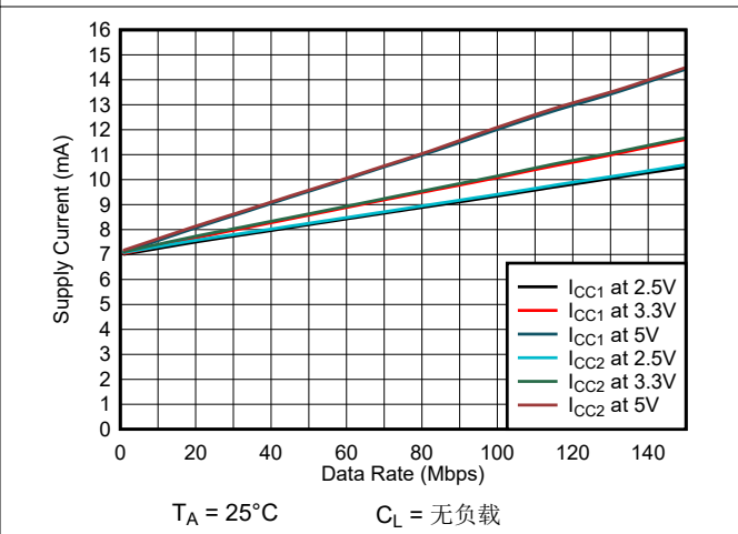
图 6-6. ISO6463 或 ISO6463F 电源电流与数据速率间的关系 (无负载)
