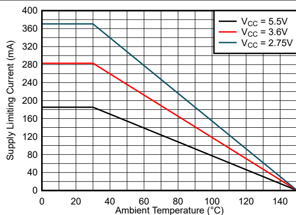
图 6-5. SSOP (DBQ-16) 封装安全限制电流的热降额曲线
