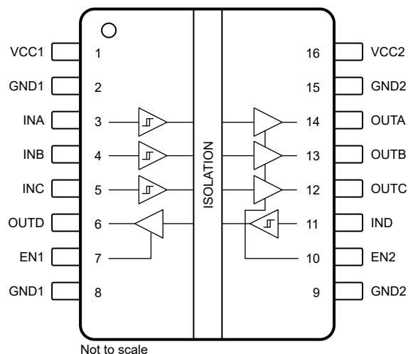
图 5-2. ISO6441-Q1 和 ISO6441F-Q1 顶视图
