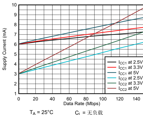
图 6-10. ISO6441-Q1 或 ISO6441F-Q1 电源电流与数据速率间的关系 (无负载)
