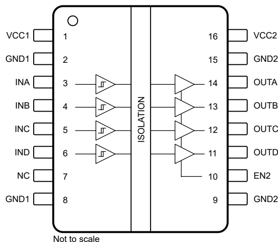
图 5-1. ISO6440-Q1 和 ISO6440F-Q1 顶视图
