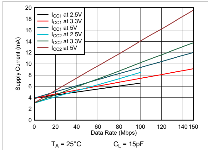
图 6-7. ISO6431-Q1 或 ISO6431F-Q1 电源电流与数据速率间的关系 (15pF 负载)
