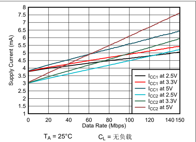
图 6-8. ISO6431-Q1 或 ISO6431F-Q1 电源电流与数据速率间的关系 (无负载)
