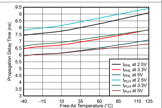
图 6-12. 传播延迟时间与自然通风条件下的温度间的关系
