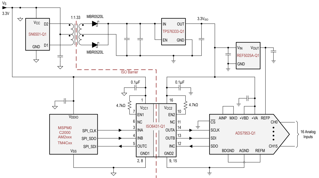
图 9-1. 3 通道典型应用
