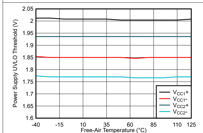
图 6-11. 电源欠压阈值与自然通风条件下的温度间的关系
