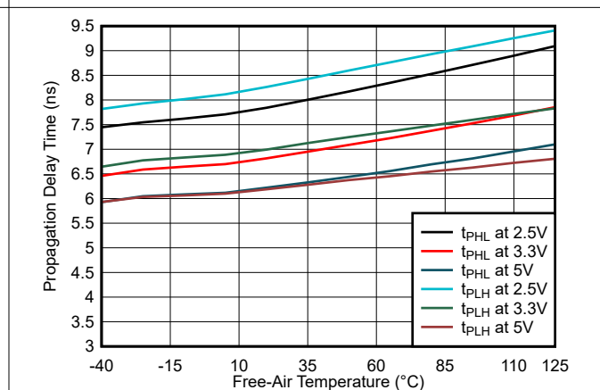
图 6-12. 传播延迟时间与自然通风条件下的温度间的关系
