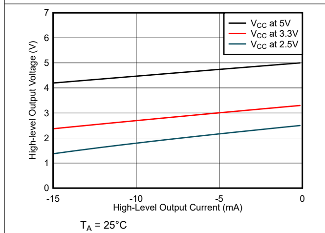
图 6-9. 高电平输出电压与高电平输出电流间的关系
