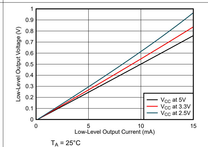
图 6-10. 低电平输出电压与低电平输出电流间的关系
