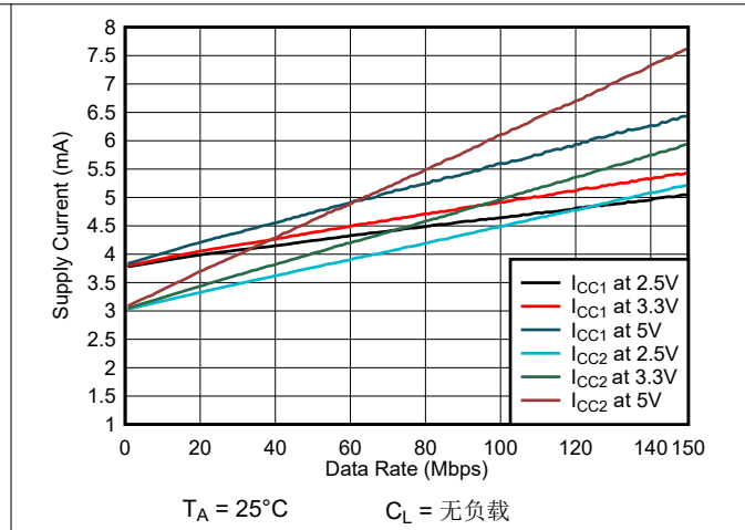
图 6-8. ISO6431 或 ISO6431F 电源电流与数据速率间的关系 (无负载)
