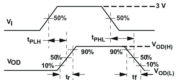
图 7-4. 驱动器开关测试电路和电压波形
