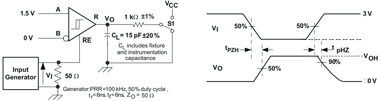
图 7-9. 接收器启用测试电路和波形，数据输出高电平
