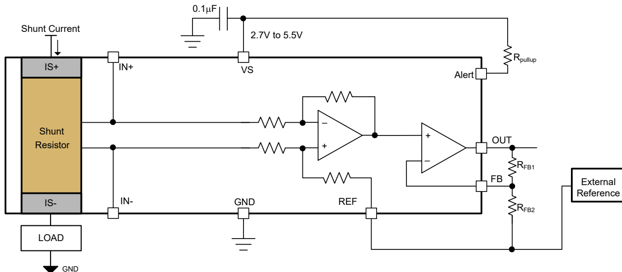
图 6-4. 调节输出
