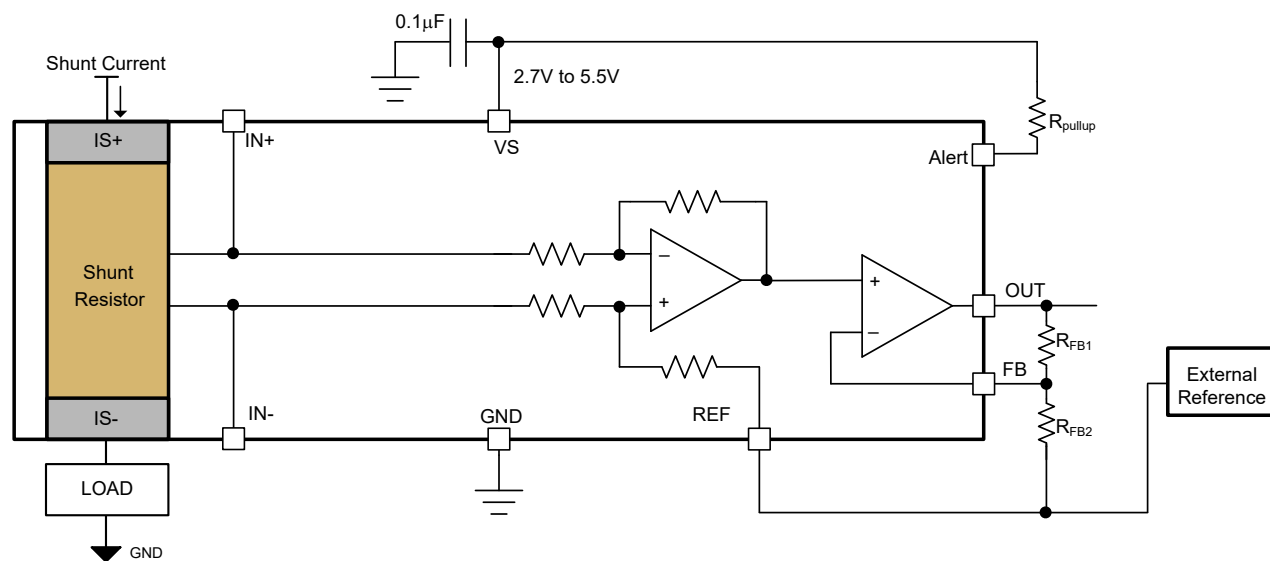
图 6-9. 热警报功能
