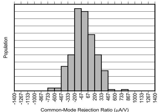
图 5-6. INA791B-Q1 共模抑制产生分布图
