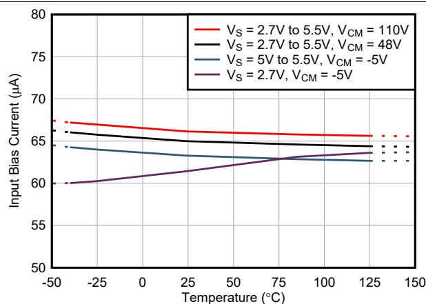
图 5-21. 总输入偏置电流与温度间的关系
