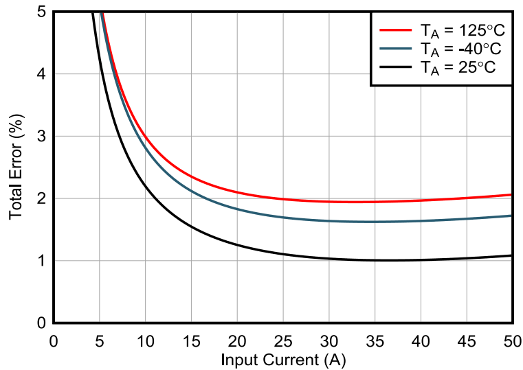
图 7-1. INA791A-Q1 总误差与输入电流间的关系
