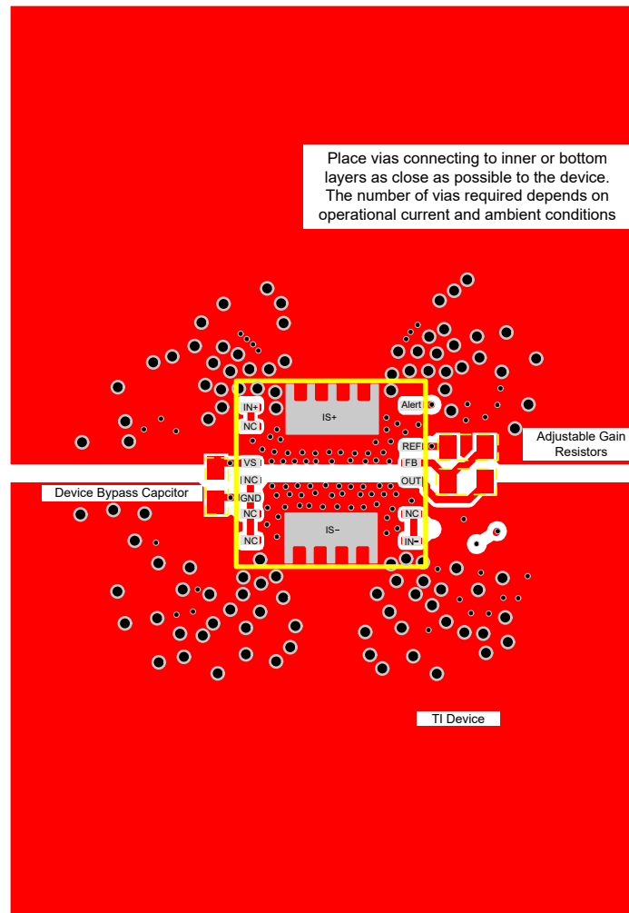
图 7-10. INA791x-Q1 布局示例
