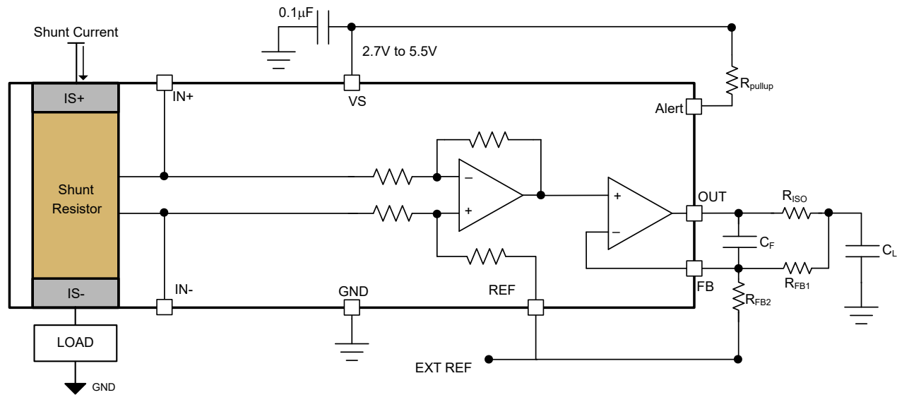
图 7-5. 具有 RISO 双反馈的 INA791x-Q1
