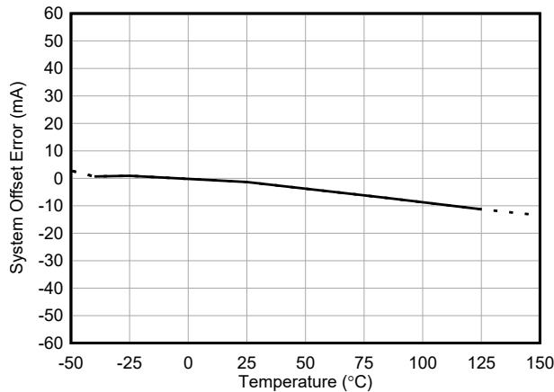
图 5-3. INA791A-Q1 输入失调电流与温度间的关系
