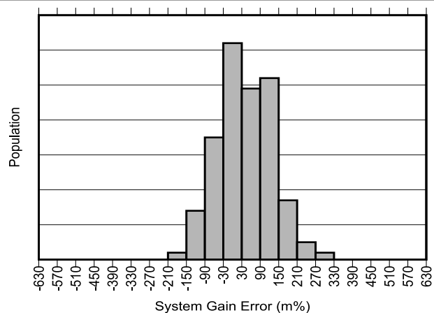
图 5-12. INA791B-Q1 增益误差产生分布图
