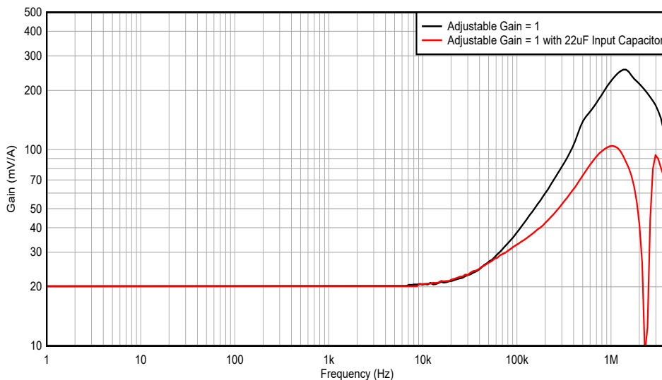
图 7-4. 添加 22μF 输入电容器之前和之后 INA791x-Q1 增益与频率间的关系
