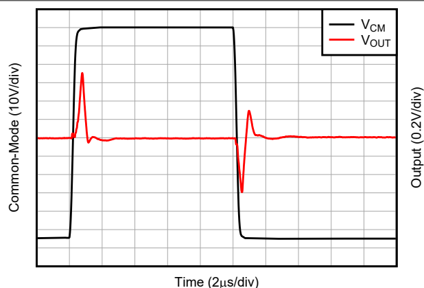
图 5-34. 共模瞬态响应
