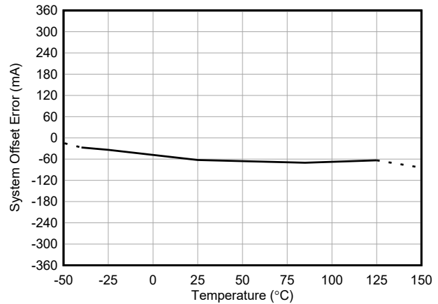
图 5-4. INA791B-Q1 输入失调电流与温度间的关系
