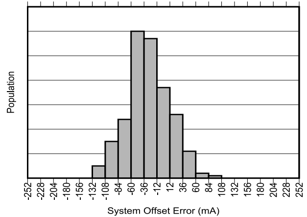
图 5-2. INA791B-Q1 输入失调电流产生分布图
