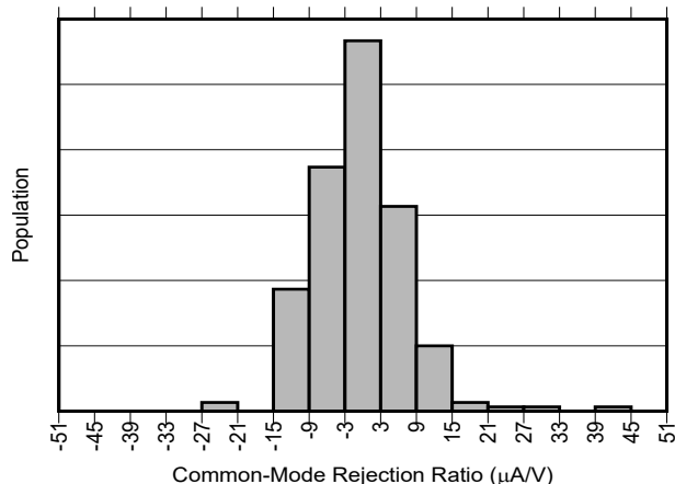
图 5-5. INA791A-Q1 共模抑制产生分布图
