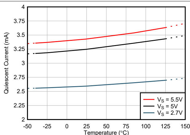
图 5-23. 静态电流与温度间的关系
