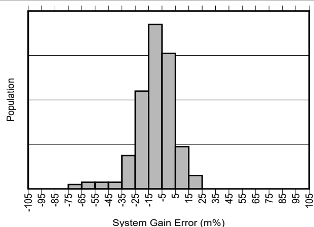
图 5-11. INA791A-Q1 增益误差产生分布图
