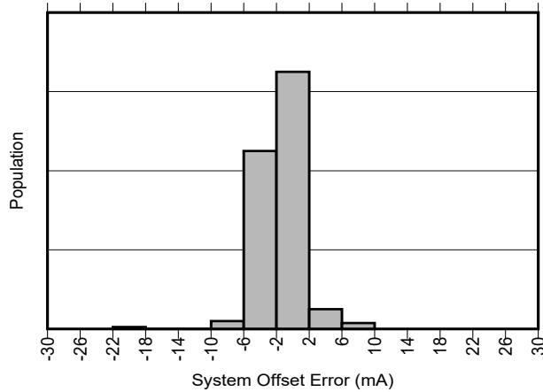
图 5-1. INA791A-Q1 输入失调电流产生分布图
