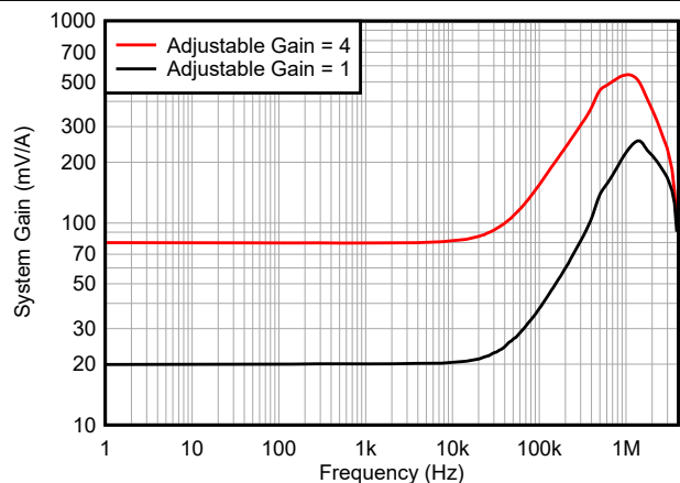
图 5-27. 系统增益与频率间的关系
