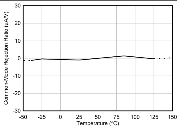
图 5-7. 共模抑制比与温度间的关系
