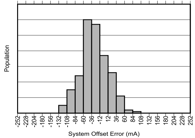
图 5-2. INA791B 输入失调电流产生分布图
