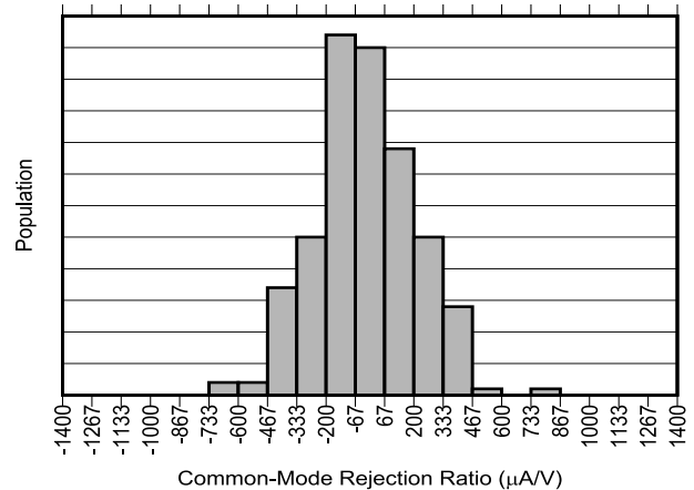
图 5-6. INA791B 共模抑制产生分布图
