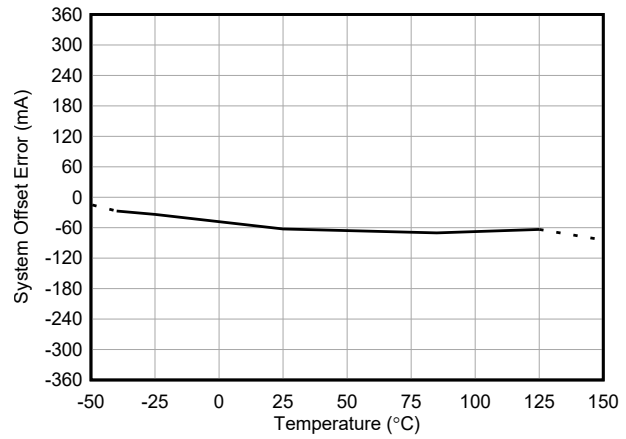
图 5-4. INA791B 输入失调电流与温度间的关系
