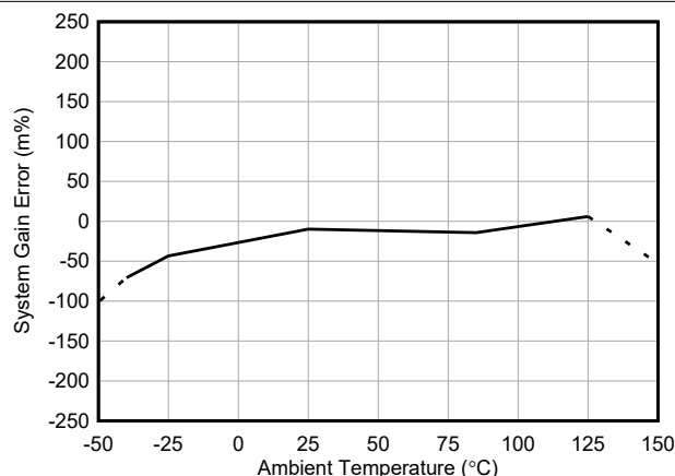
图 5-13. INA790A-Q1 增益误差与温度间的关系
