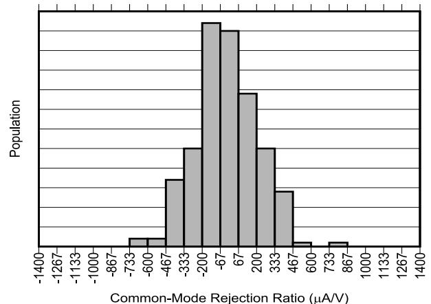
图 5-6. INA790B-Q1 共模抑制产生分布图
