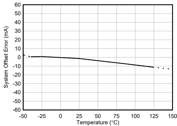
图 5-3. INA790A-Q1 输入失调电流与温度间的关系
