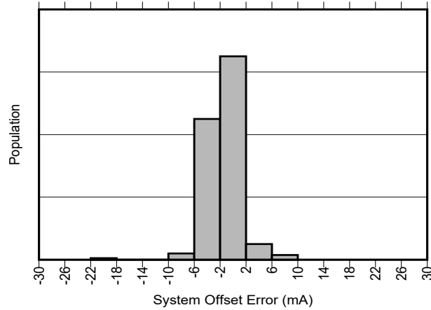
图 5-1. INA790A-Q1 输入失调电流产生分布图
