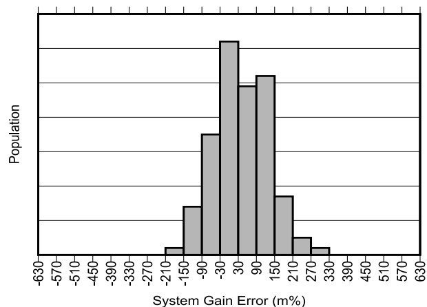
图 5-12. INA790B-Q1 增益误差产生分布图
