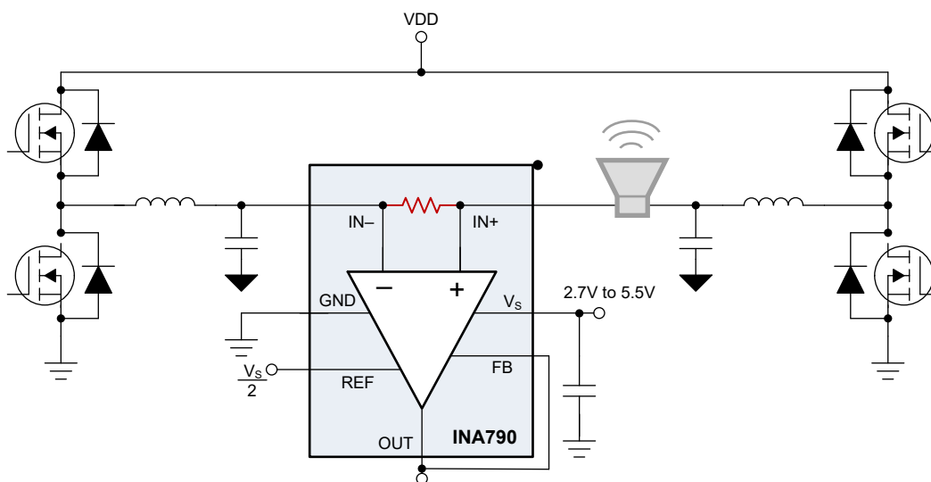
图 7-10. D 类系统中的电流检测
