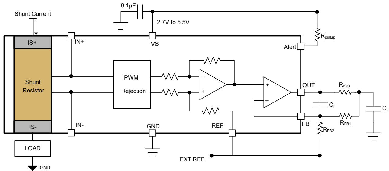
图 7-5. 具有 RISO 双反馈的 INA790x-Q1
