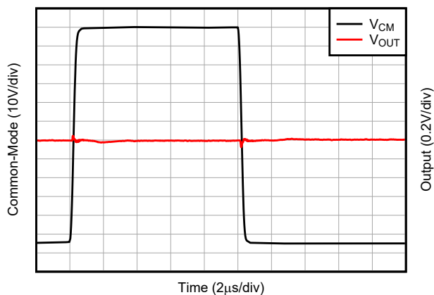
图 5-34. -4V 至 110V 共模阶跃瞬态响应
