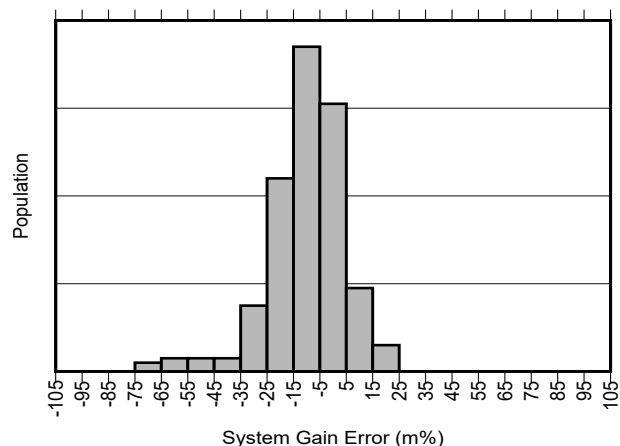
图 5-11. INA790A-Q1 增益误差产生分布图
