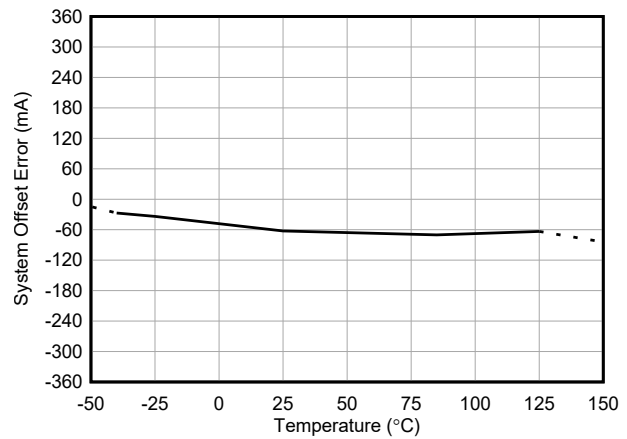
图 5-4. INA790B-Q1 输入失调电流与温度间的关系
