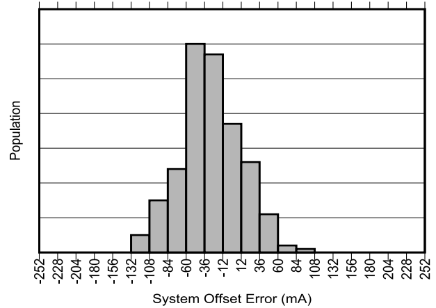
图 5-2. INA790B-Q1 输入失调电流产生分布图
