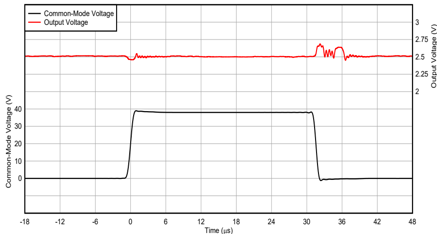
图 6-4. 增强型 PWM 抑制性能
