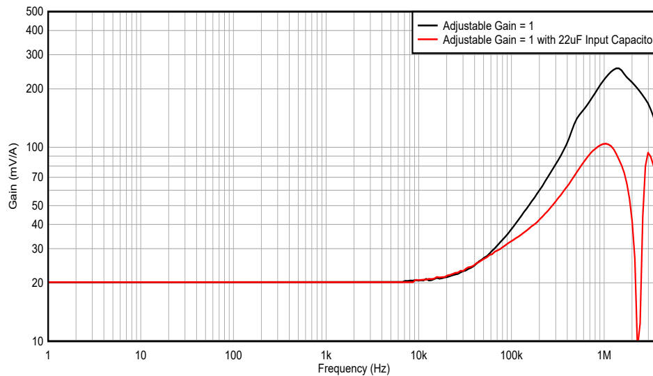
图 7-4. 添加 22μF 输入电容器之前和之后 INA790x-Q1 增益与频率间的关系
