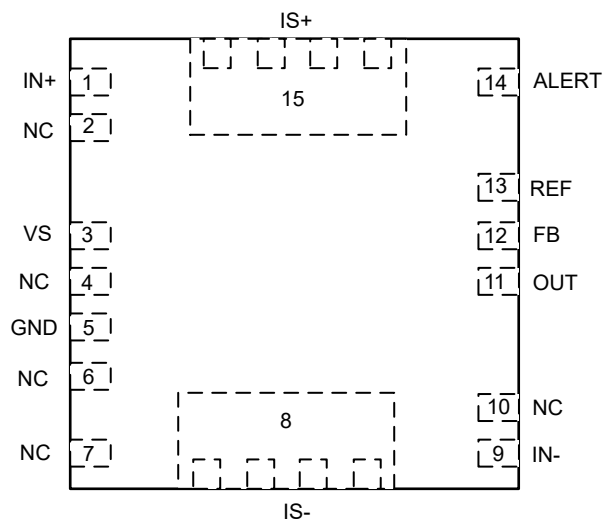
图 4-1. INA790x-Q1 可湿性 DEK 封装 15 引脚 VQFN 顶视图
