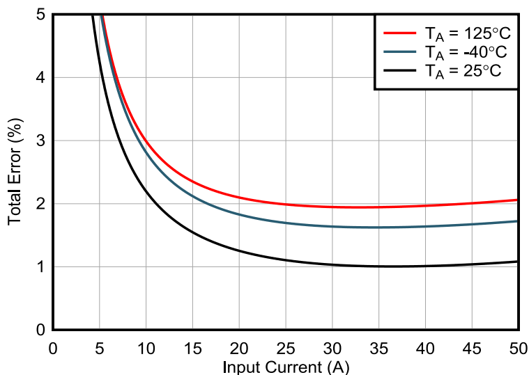
图 7-1. INA790A-Q1 总误差与输入电流间的关系
