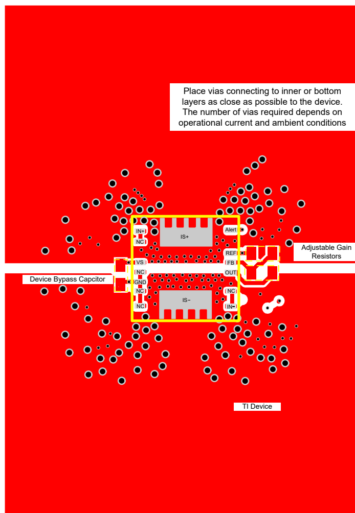
图 7-12. INA790x-Q1 布局示例
