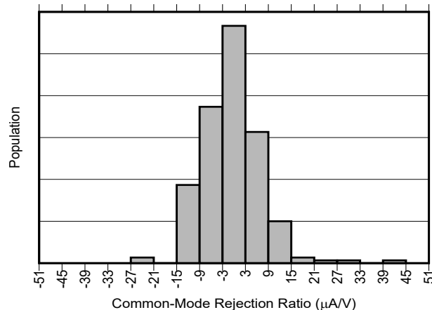
图 5-5. INA790A-Q1 共模抑制产生分布图
