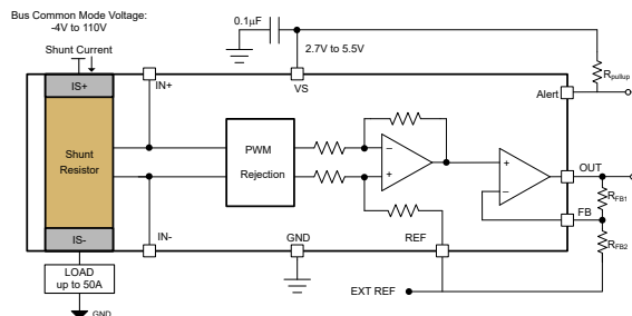
典型应用
