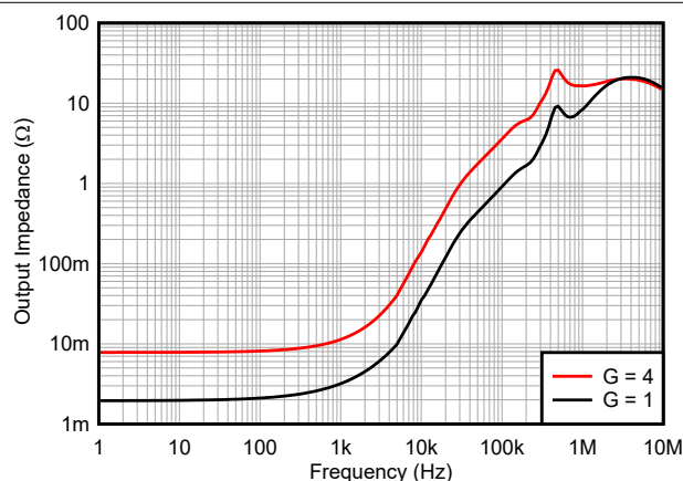
图 5-30. 输出阻抗与频率间的关系
