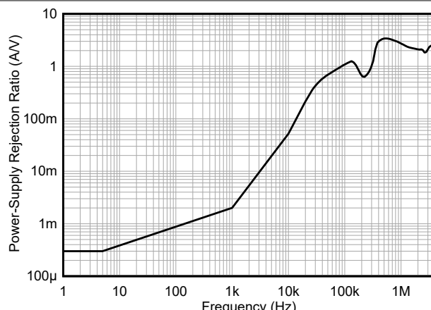
图 5-28. 电源抑制比与频率间的关系
