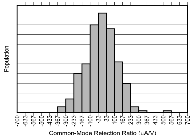
图 5-6. INA751B 共模抑制产生分布图
