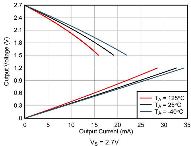
图 5-15. 输出电压摆幅与输出电流间的关系
