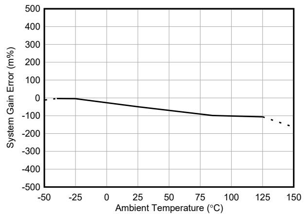
图 5-14. INA751B 增益误差与温度间的关系
