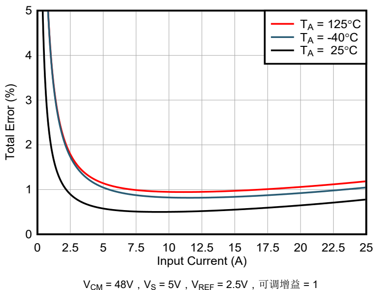
图 7-1. INA751A 总误差与输入电流间的关系
