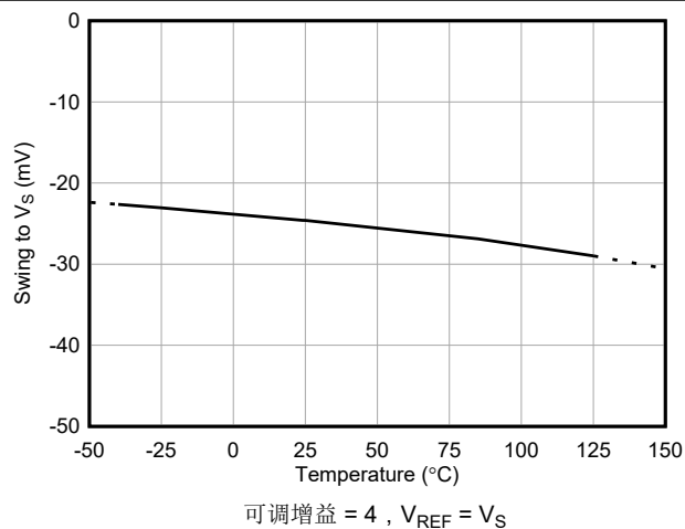
图 5-17. 输出电压摆幅高位与温度间的关系
