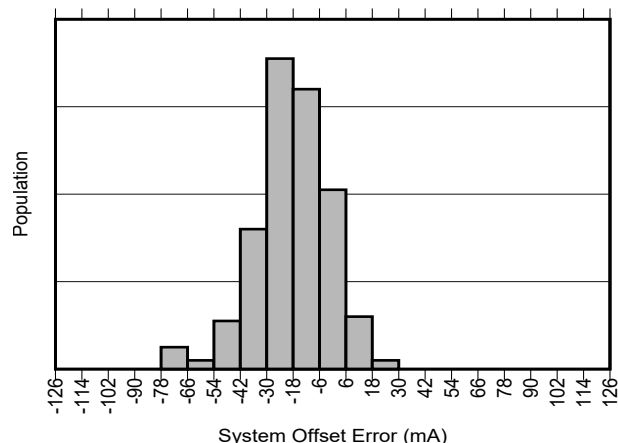
图 5-2. INA751B 输入失调电流产生分布图
