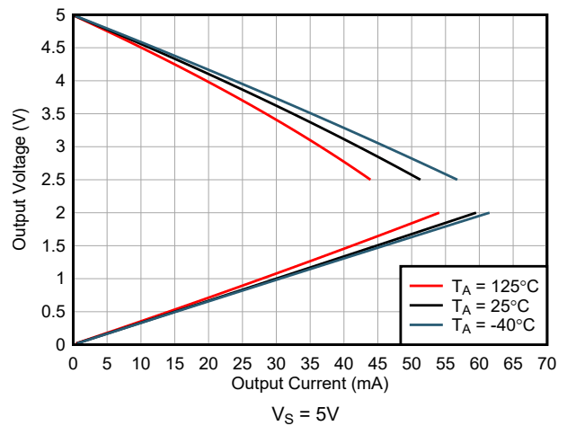
图 5-16. 输出电压摆幅与输出电流间的关系
