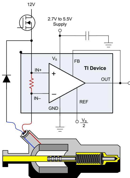
图 7-3. 螺线管驱动应用电路
