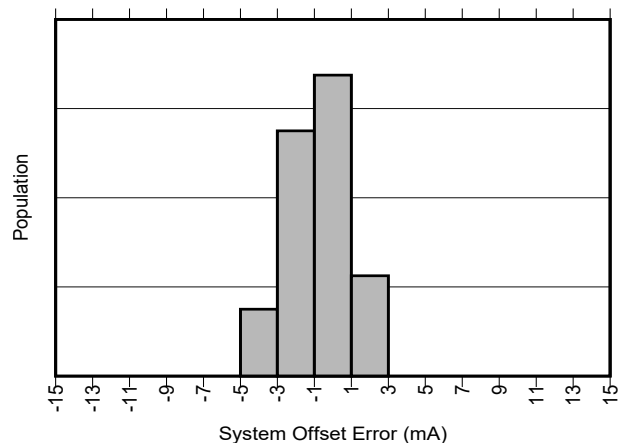
图 5-1. INA751A 输入失调电流产生分布图
