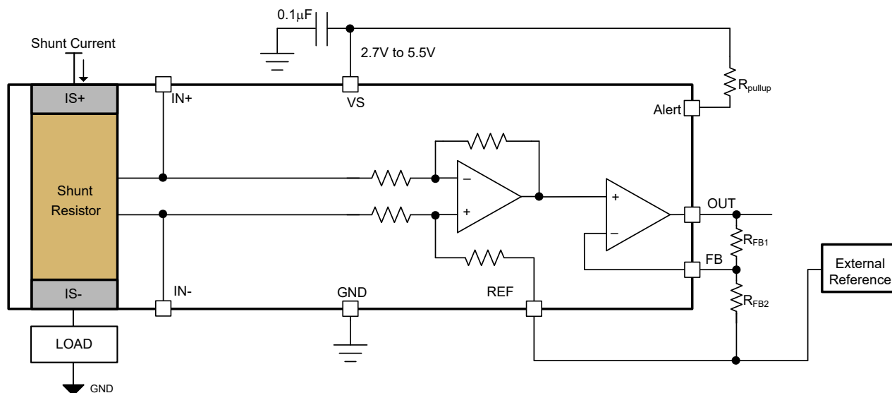
图 6-4. 调节输出
