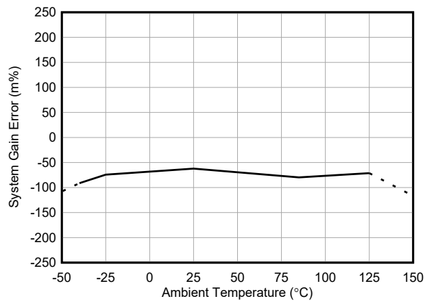
图 5-13. INA751A 增益误差与温度间的关系
