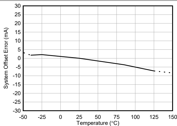
图 5-3. INA751A 输入失调电流与温度间的关系
