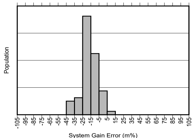
图 5-11. INA751A 增益误差产生分布图
