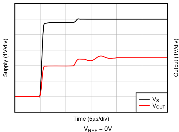
图 5-35. 启动响应
