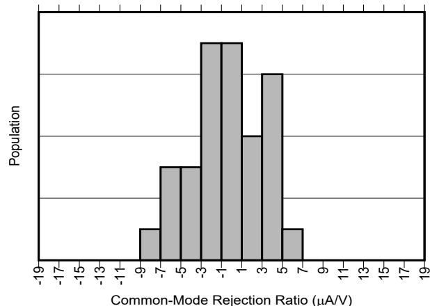
图 5-5. INA751A 共模抑制产生分布图
