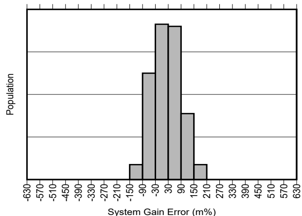
图 5-12. INA751B 增益误差产生分布图
