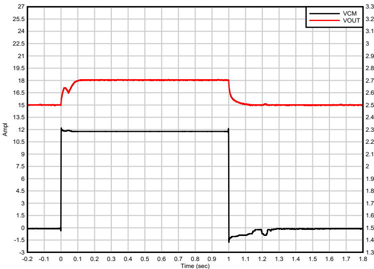
图 7-4. 螺线管驱动电流检测输入和输出信号
