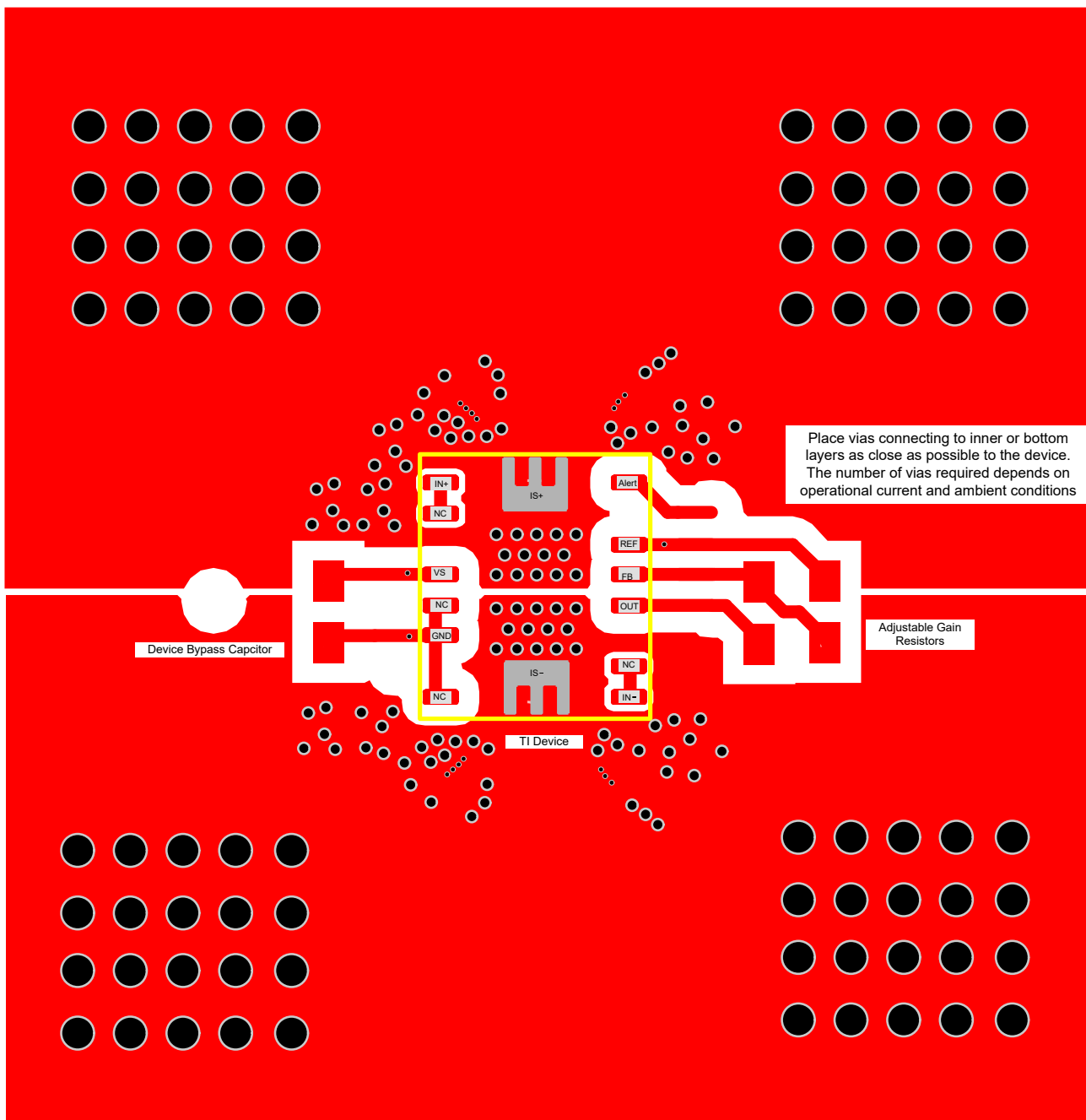
图 7-5. INA751x 布局示例
