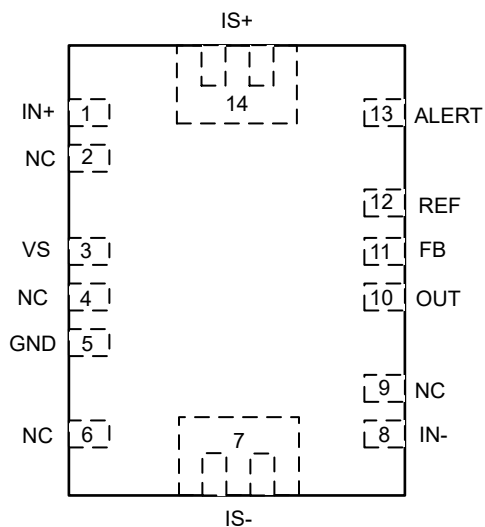
图 4-1. INA751x REM 封装 VQFN 顶视图
