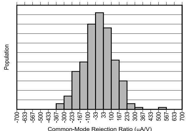
图 5-6. INA750B 共模抑制产生分布图
