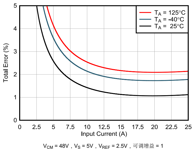
图 7-1. INA750A 总误差与输入电流间的关系
