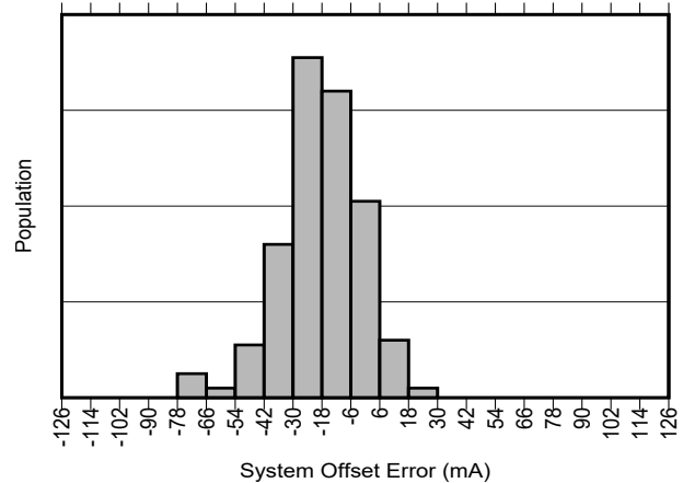
图 5-2. INA750B 输入失调电流产生分布图
