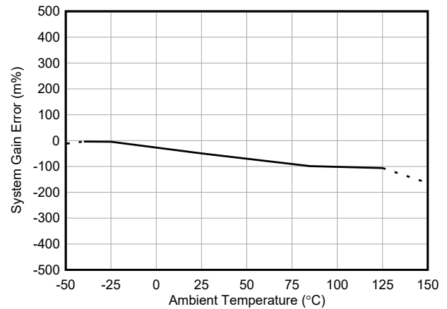
图 5-14. INA750B 增益误差与温度间的关系
