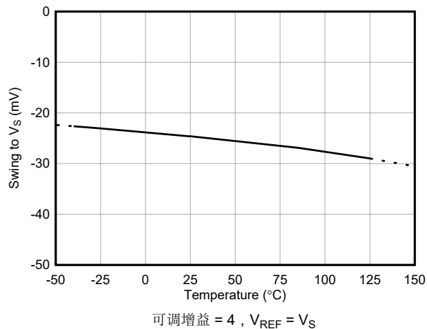
图 5-17. 输出电压摆幅高位与温度间的关系
