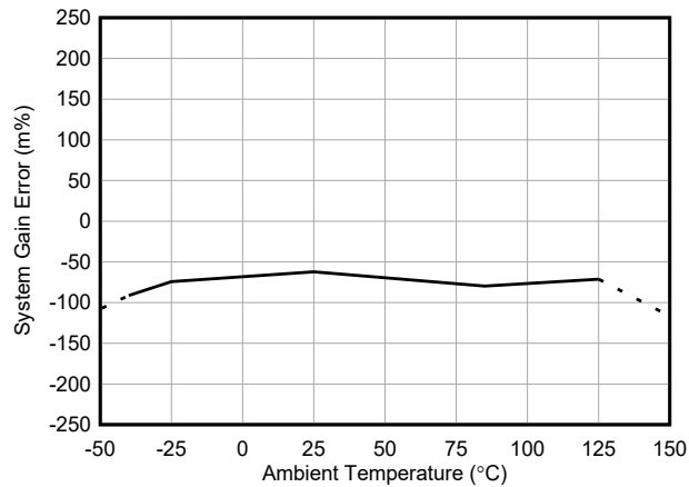
图 5-13. INA750A 增益误差与温度间的关系
