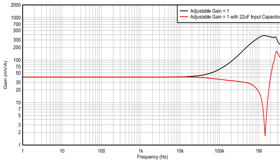
图 7-4. 添加 22μF 输入电容器之前和之后 INA750x 增益与频率间的关系
