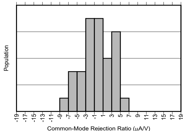
图 5-5. INA750A 共模抑制产生分布图
