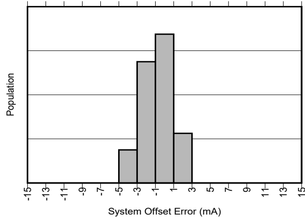
图 5-1. INA750A 输入失调电流产生分布图
