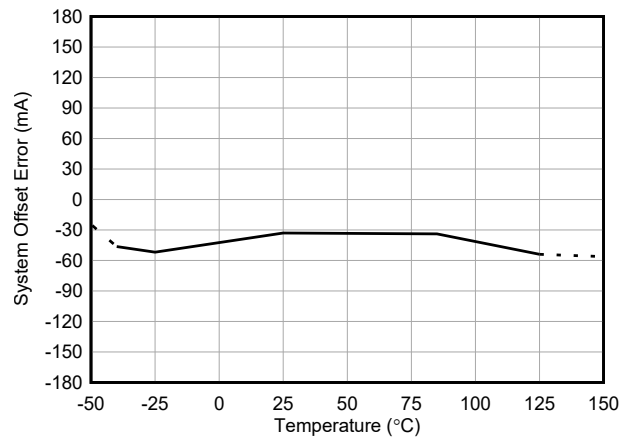
图 5-4. INA750B 输入失调电流与温度间的关系
