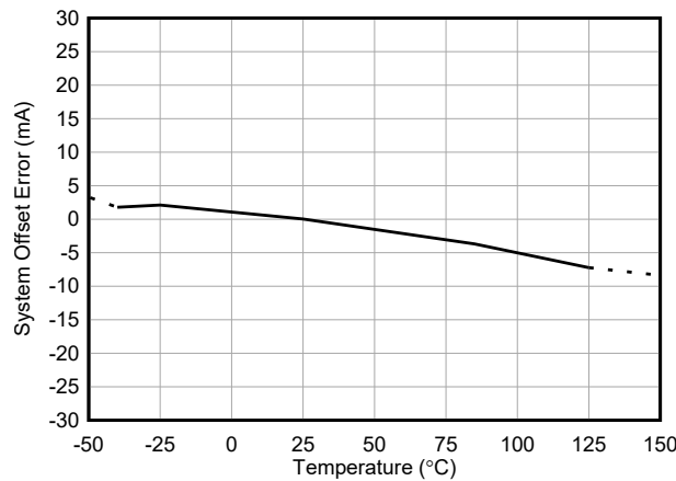
图 5-3. INA750A 输入失调电流与温度间的关系
