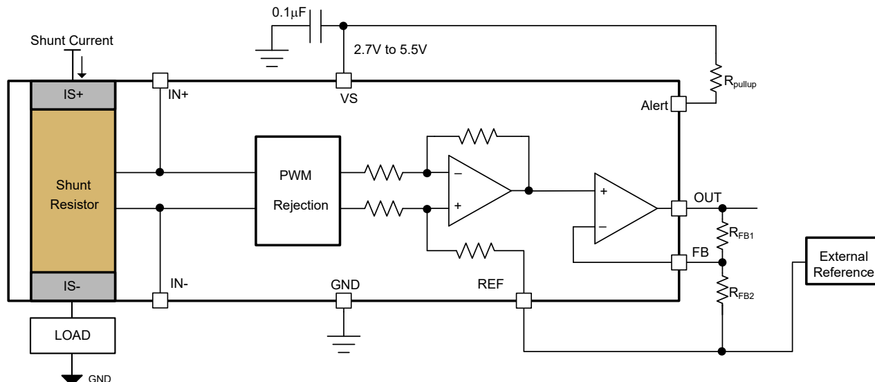
图 6-5. 调节输出
