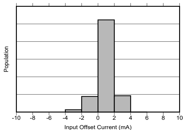
图 5-2. 分流输入偏移电流产生分布图
