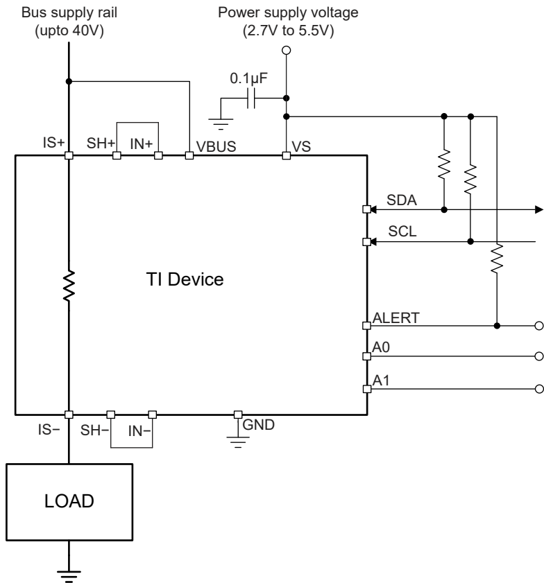
图 8-2. INA745x 高侧感测应用图
