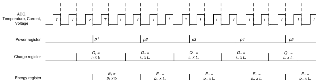
图 6-7. 功率、电能和电荷计算方案
