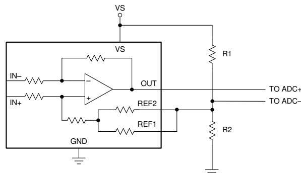
图 7-8. 使用电阻分压器设置基准
