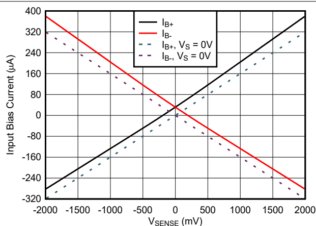
图 6-18. INA241x-Q1 输入偏置电流与 V_{\text{SENSE}} 间的关系
