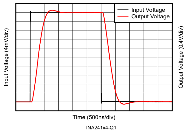
图 6-35. 大阶跃响应
