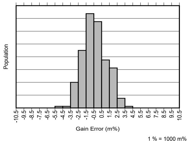
图 6-11. INA241A4-Q1 和 增益误差产生分布图
