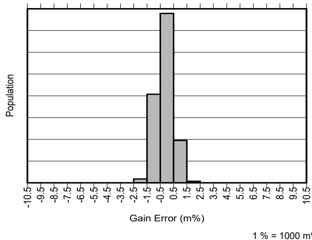
图 6-10. INA241A1-Q1, INA241A2-Q1, INA241A3-Q1 增益误差产生分布图
