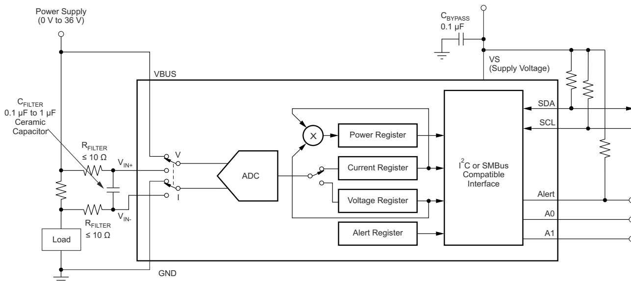
图 8-3. Input Filtering
