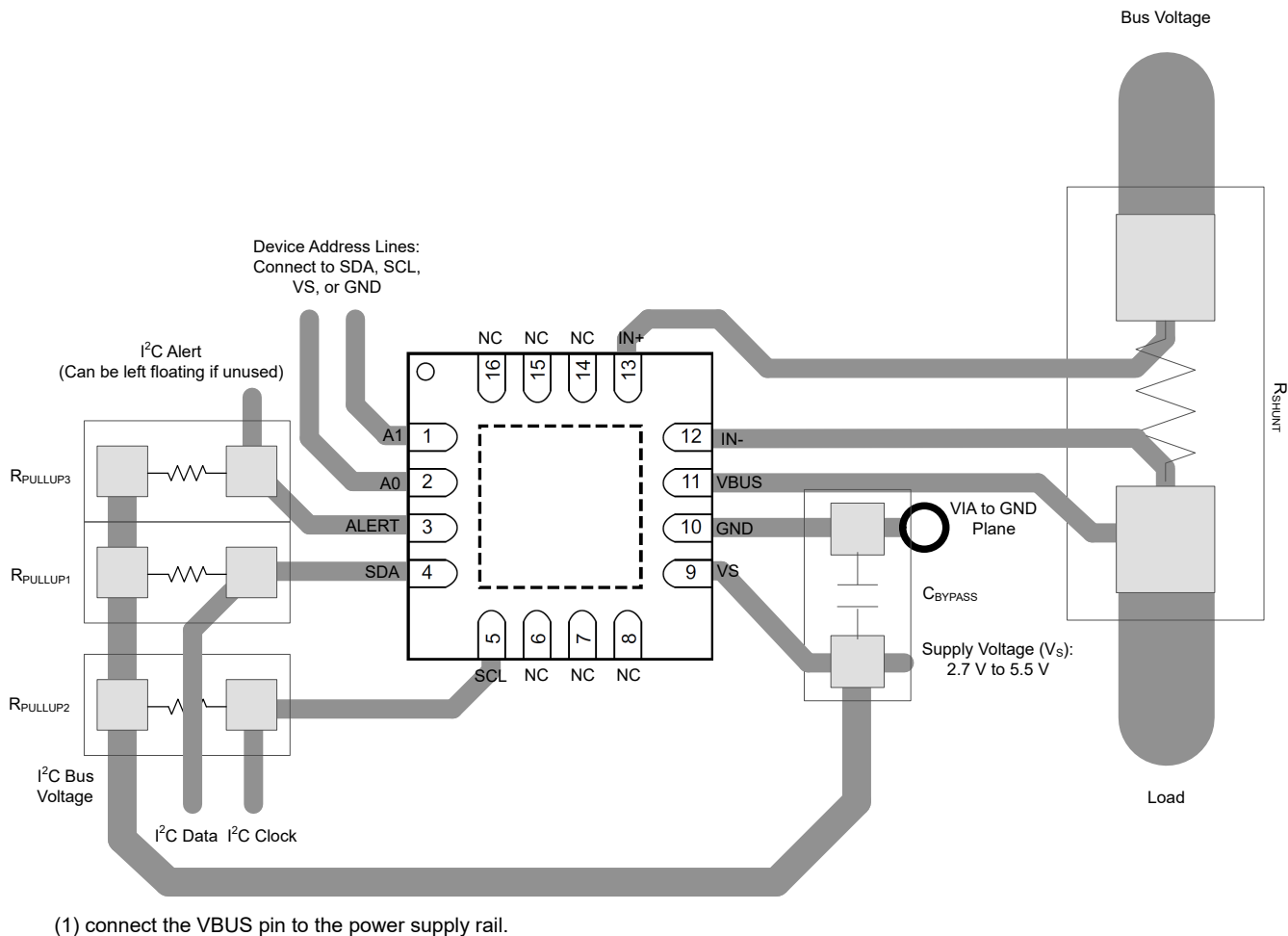
图 11-1. Layout Example (RGT Package)
