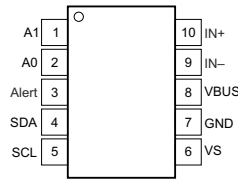
图 6-2. DGS Package 10-Pin VSSOP (Top View)
