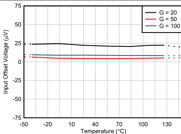
图 5-2. 输入失调电压与温度间的关系
