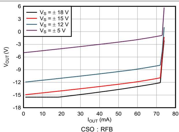
图 5-10. 最大 V_{\text{OUT}} 与 I_{\text{OUT}} 间的关系 (正摆幅)
