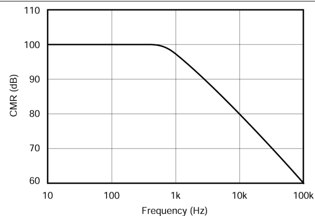
图 5-11. CMR 与频率间的关系
