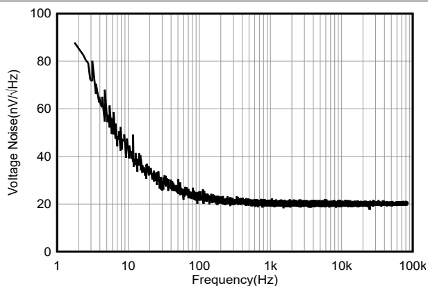
图 5-14. 电压噪声密度与频率间的关系
