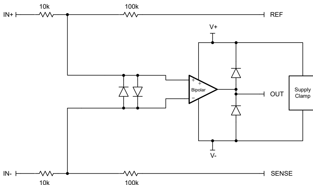
图 6-1. 以下制造过程的 INA106 内部原理图：CSO: SHE
