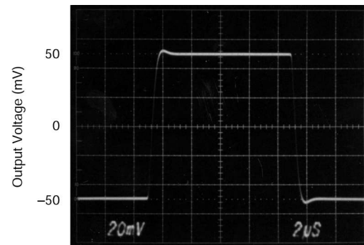
2 μs/div 图 5-4. 微小信号响应 ( R_{\text{LOAD}} = \infty , C_{\text{LOAD}} = 100\text{pF} )
