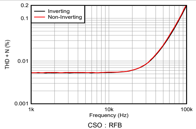
图 5-6. 总谐波失真和噪声与频率间的关系
