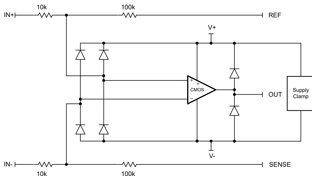
图 6-2. 以下制造过程的 INA106 内部原理图：CSO: RFB
