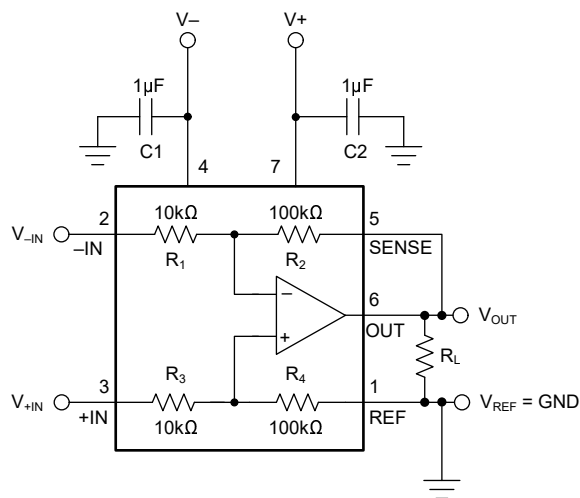
图 7-9. 示例原理图
