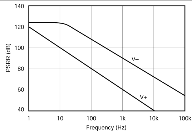
图 5-12. 电源抑制与频率间的关系
