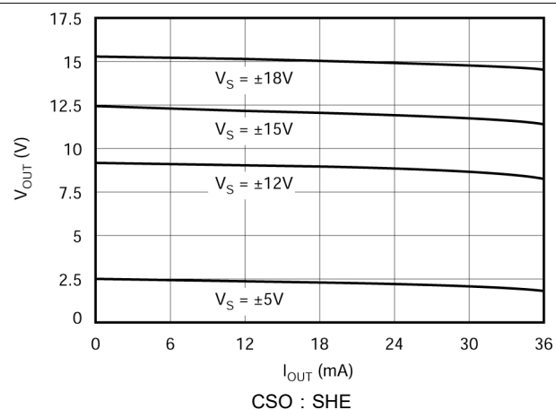
图 5-9. 最大 V_{\text{OUT}} 与 I_{\text{OUT}} 间的关系 (正摆幅)
