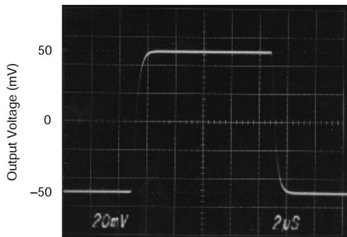
2 μs/div 图 5-3. 微小信号响应 (空载)
