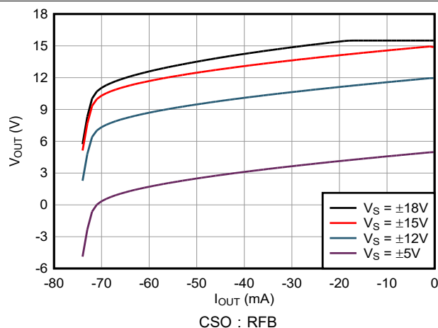
图 5-8. 最大 V_{\text{OUT}} 与 I_{\text{OUT}} 间的关系 (负摆幅)
