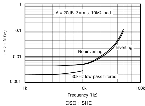
图 5-5. 总谐波失真和噪声与频率间的关系
