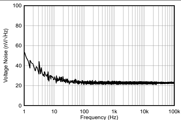
图 5-13. 电压噪声密度与频率间的关系
