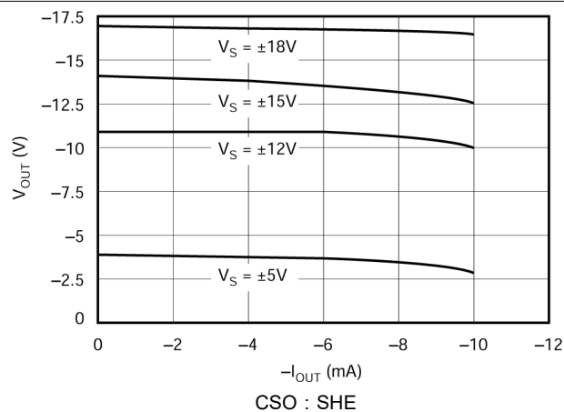
图 5-7. 最大 V_{\text{OUT}} 与 I_{\text{OUT}} 间的关系 (负摆幅)
