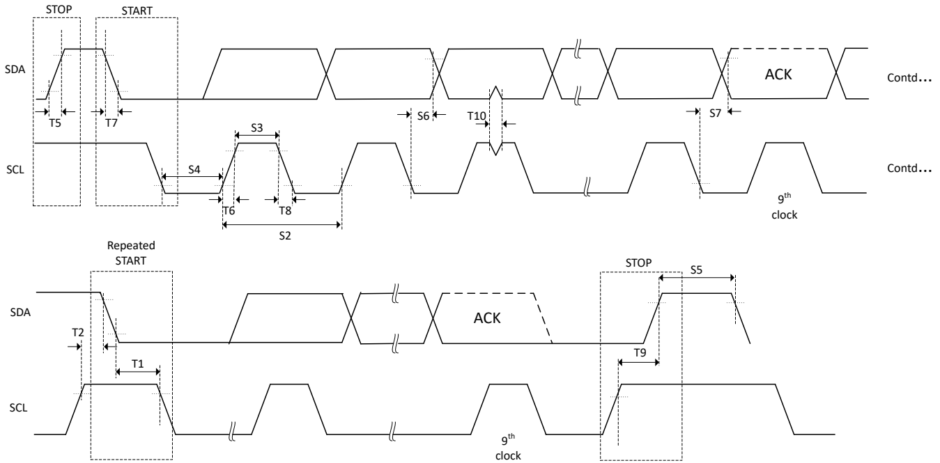
图 6-60. I2C 时序图
