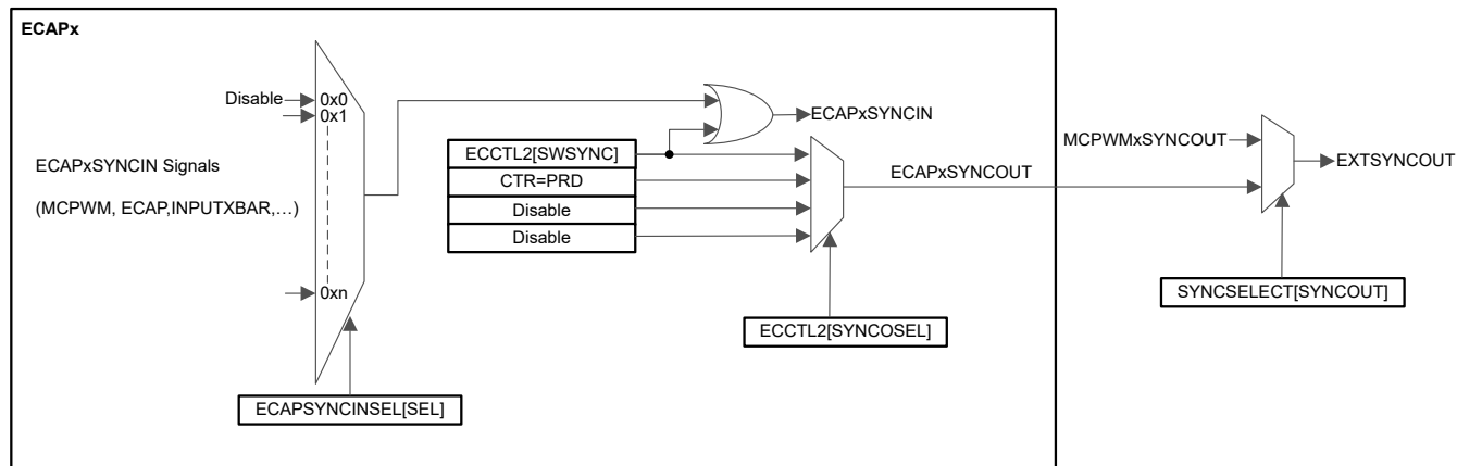
图 6-58. eCAP 同步方案
