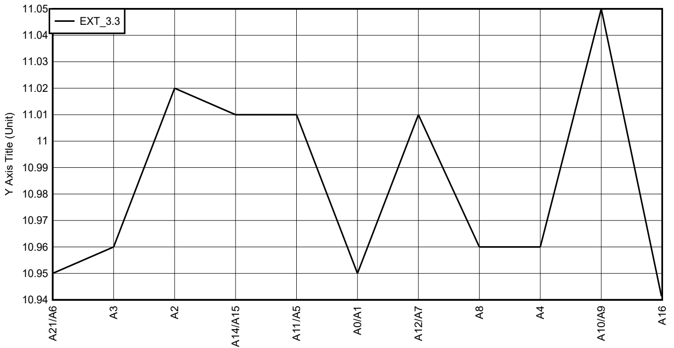
图 6-39. 32 引脚 RHB 的每通道 ENOB
