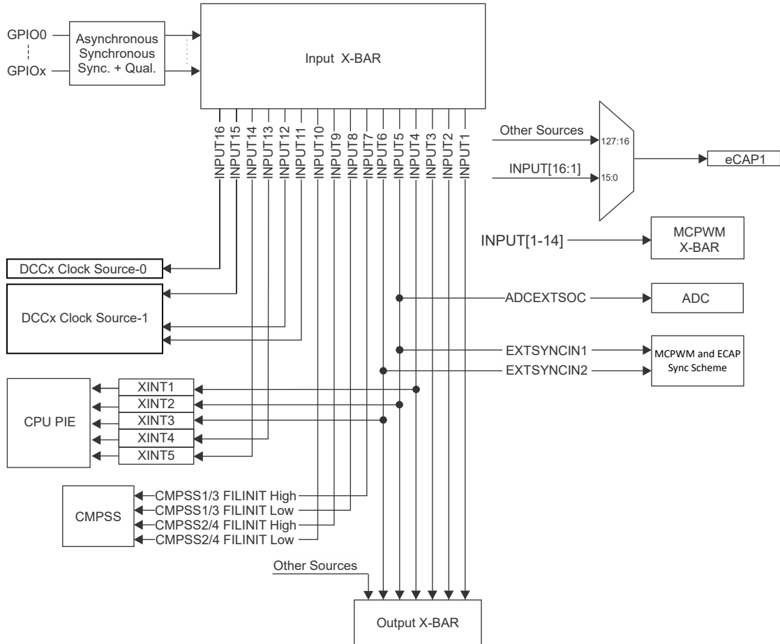
图 5-4. 输入 X-BAR
