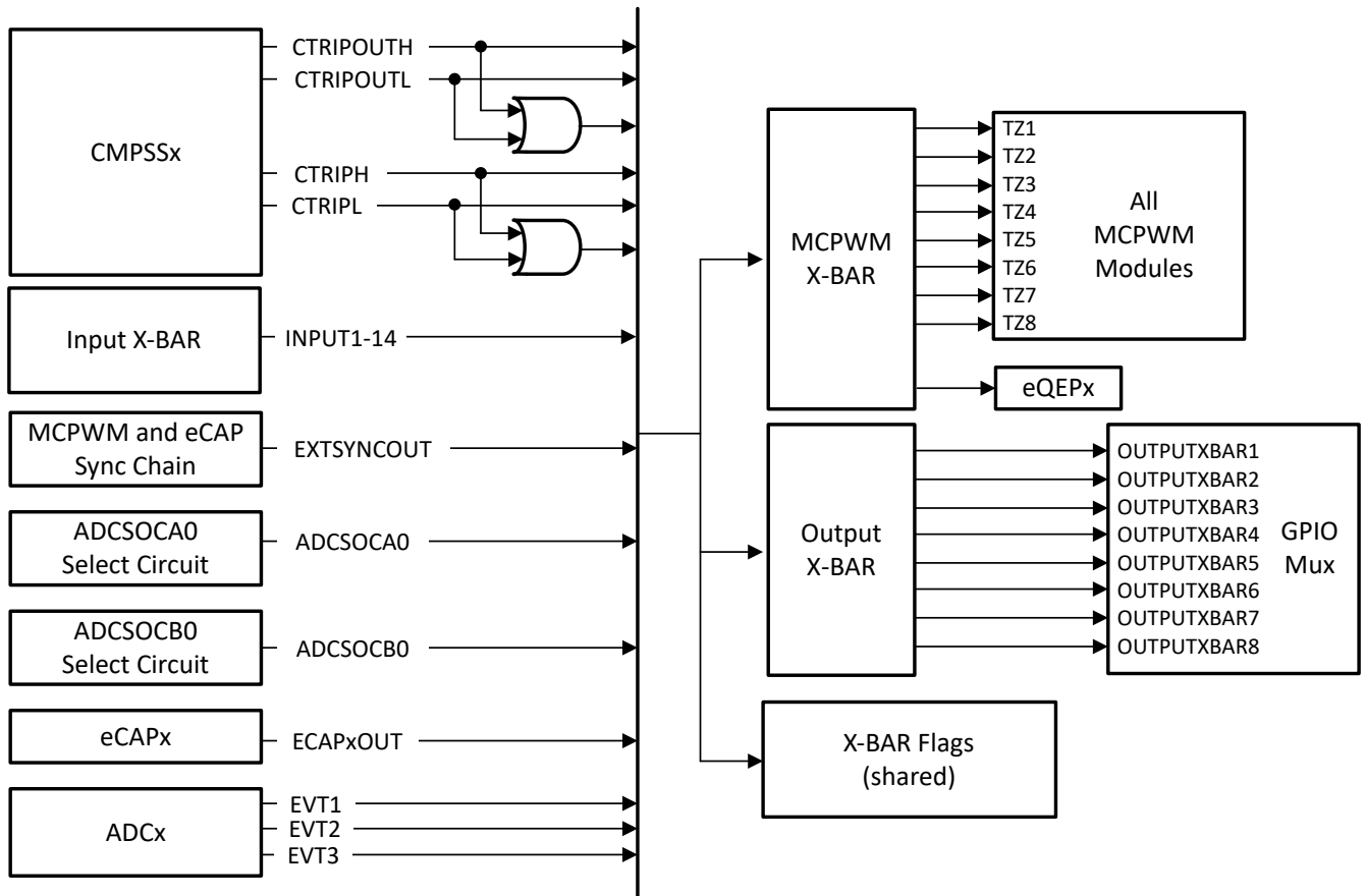
图 5-5. GPIO 输出 X-BAR 和 PWM X-BAR 源
