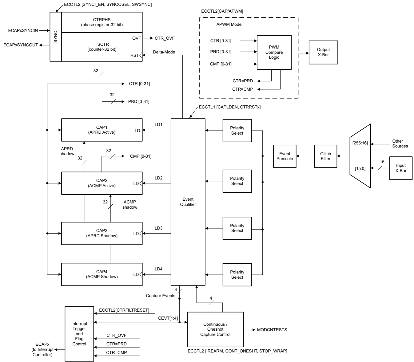
图 6-57. eCAP 方框图
