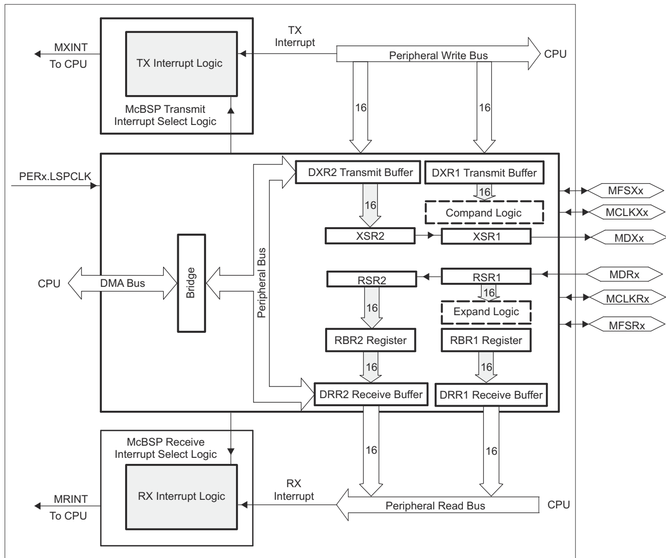
图 6-66. McBSP 方框图
