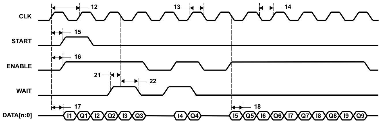
图 6-85. uPP 双倍数据速率 (DDR) 发送时序
