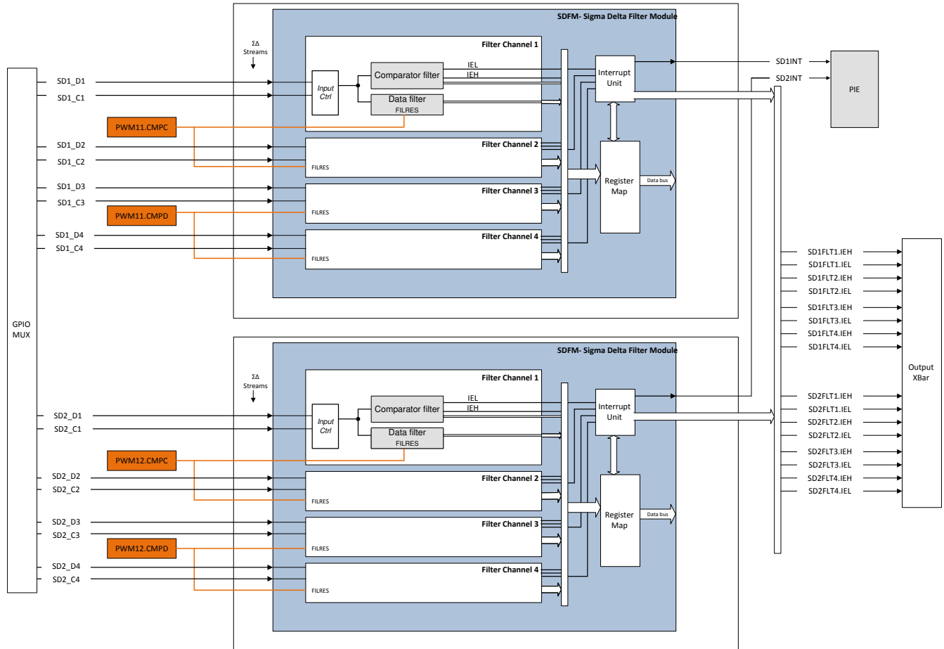
图 6-58. SDFM 方框图
