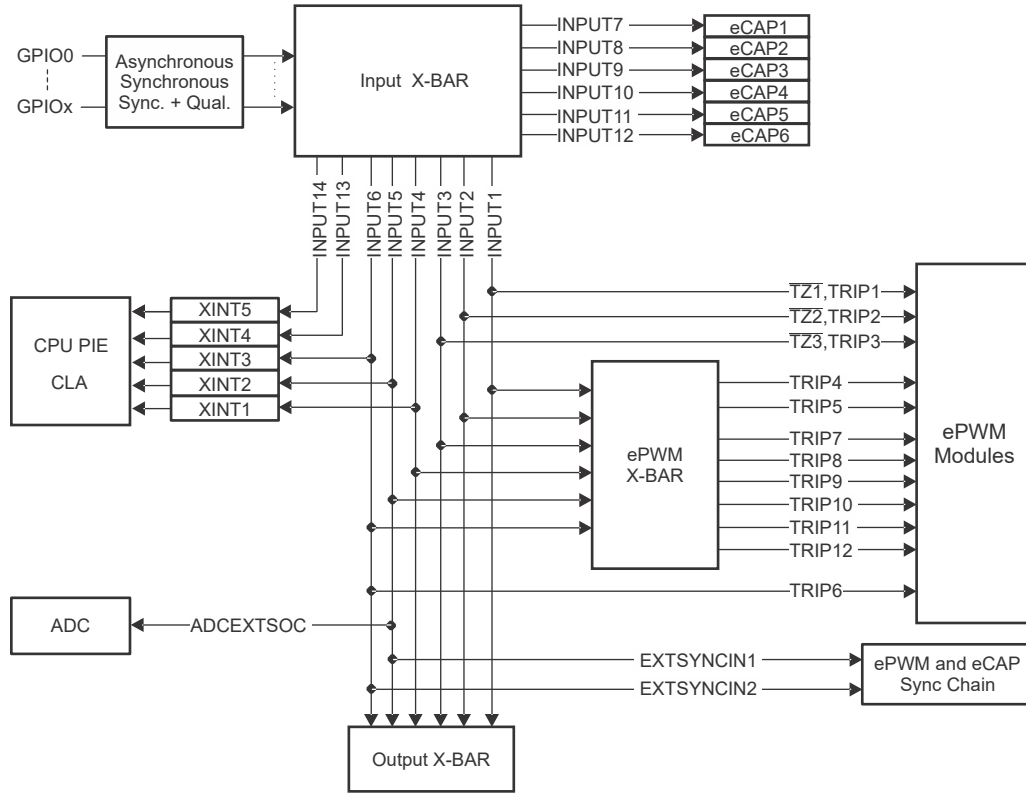
图 5-2. 输入 X-BAR
