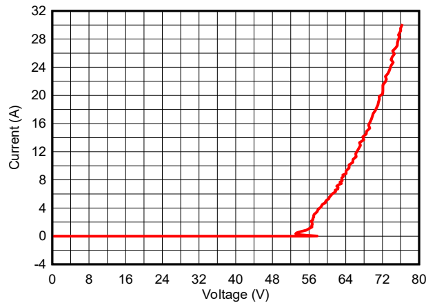
图 5-3. 正 TLP 曲线
