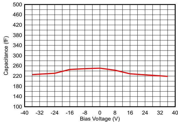
图 5-1. 偏置电压与电容间的关系
