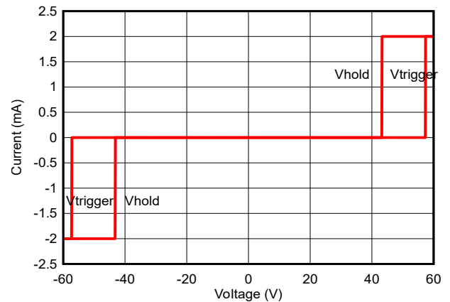
图 5-2. 直流 I-V 曲线
