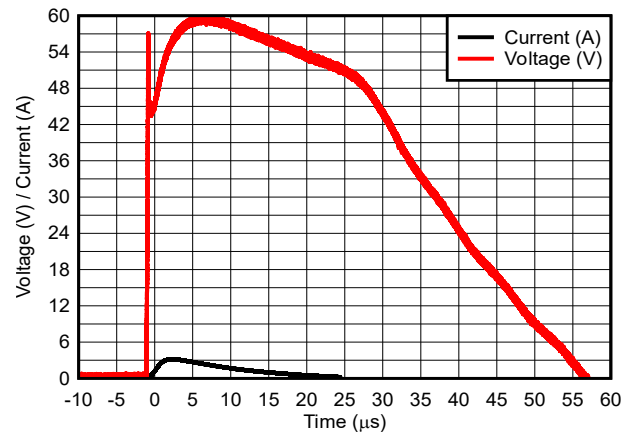
图 5-4. 8/20 \mu\text{s} 浪涌响应
