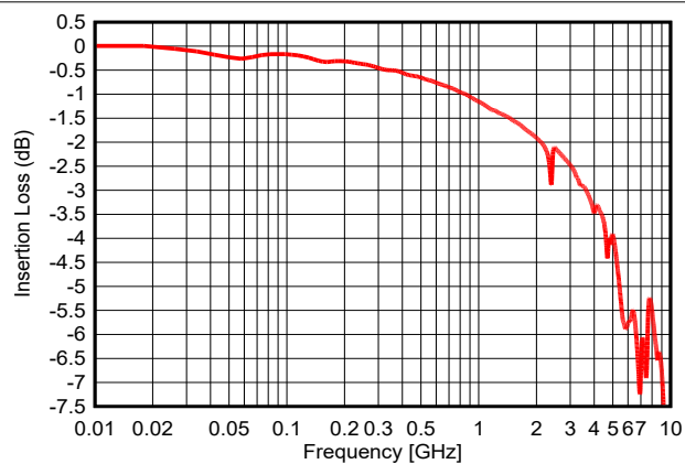
图 5-8. 插入损耗
