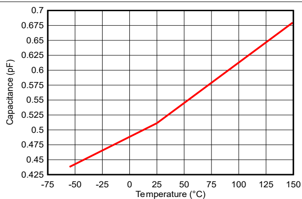
图 5-6. 电容与温度间的关系
