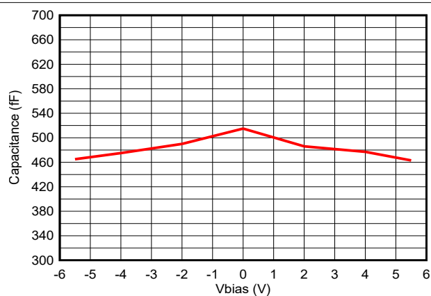
图 5-5. 电容与偏置电压之间的关系
