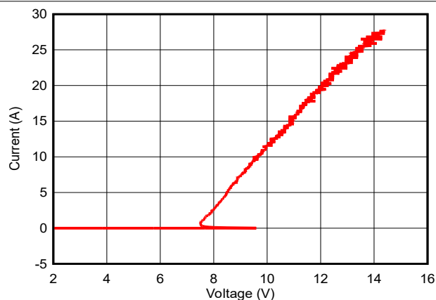
图 5-1. 正 TLP 曲线
