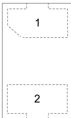
图 4-1. DPY 封装，2 引脚 DFN1006 ( 顶视图 )
