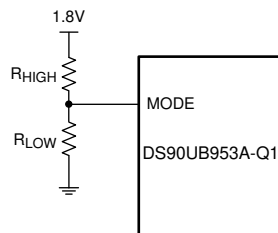
图 6-7. MODE 配置
