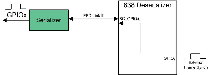
图 7-10. External FrameSync
