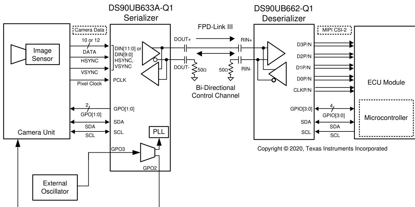
图 7-4. DS90UB633A-Q1/662-Q1 Operation in the External Oscillator Mode
