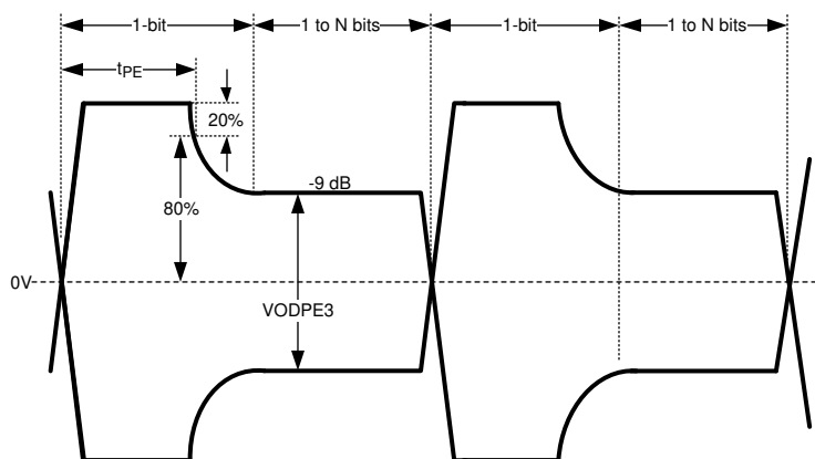
图 5-3. 输出预加重持续时间的测试条件
