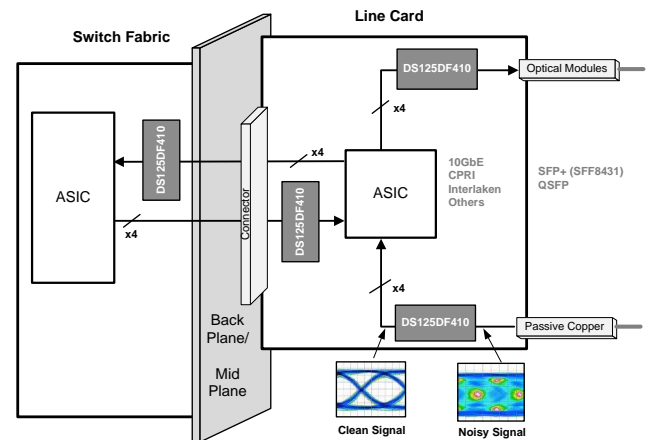
典型应用图
