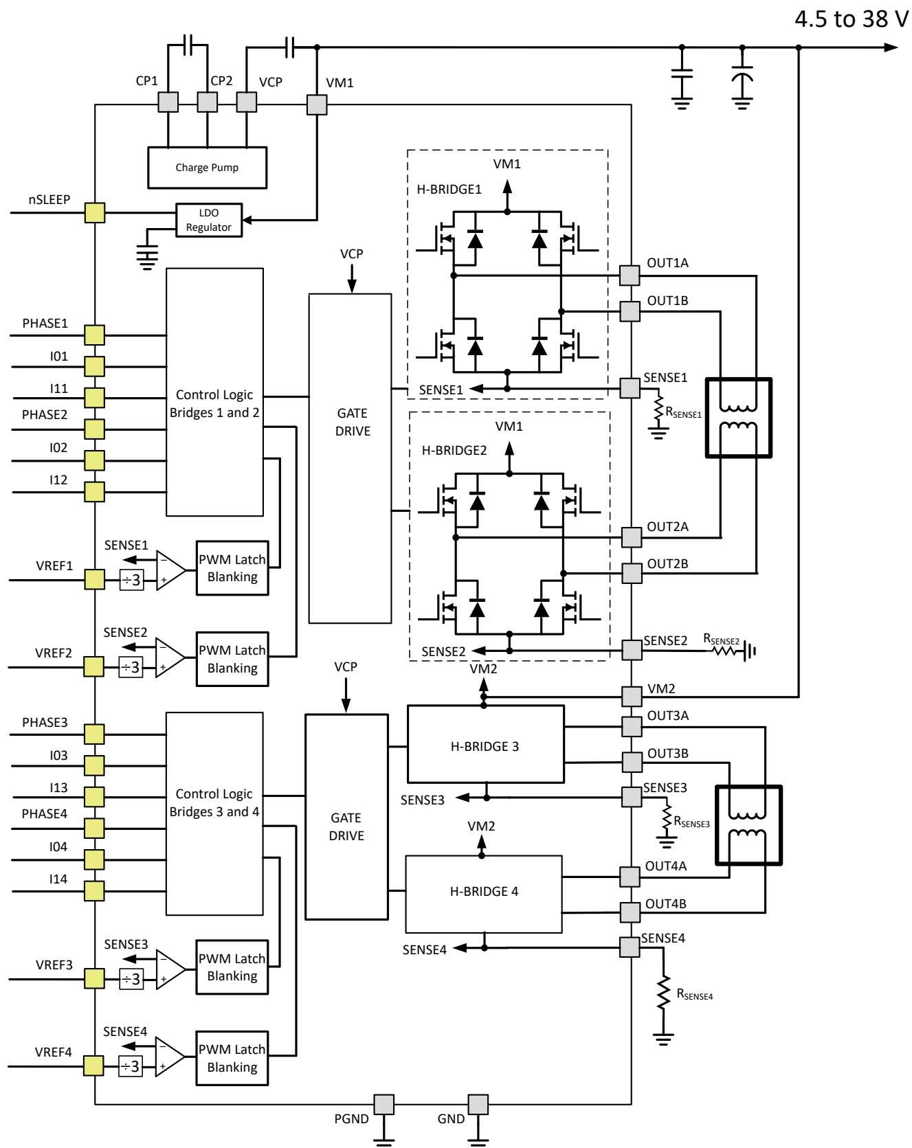
图 7-1. 功能方框图
