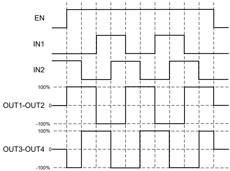
图 7-6. 全步进模式
