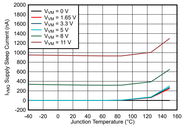
A. V_{VCC} = 3.3\text{V} 图 7-2. 休眠电流 ( I_{VMQ} ) 与结温 ( T_J )
