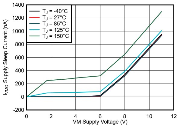
A. V_{VCC} = 3.3\text{V} 图 7-1. 休眠电流 ( I_{VMQ} ) 与电源电压 ( V_{VM} )
