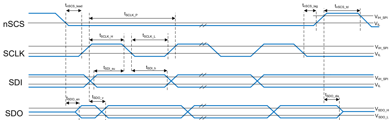
图 5-1. SPI 时序图
