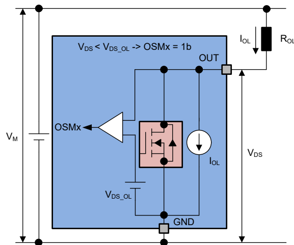
图 6-14. 输出状态监控
