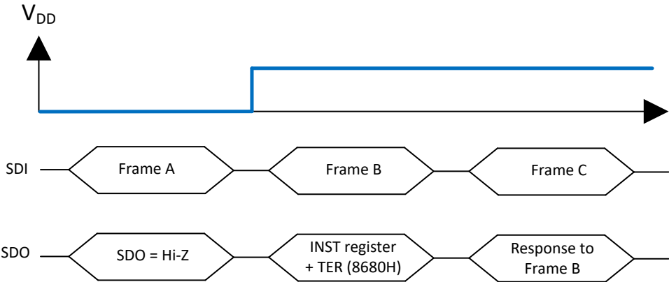
图 6-20. 退出 V_{DD} 上电复位后的响应
