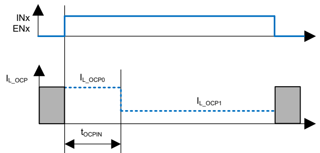
图 6-10. 过流阈值
