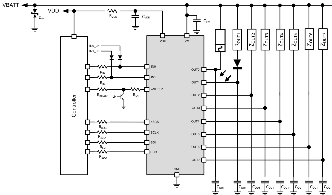
图 7-1. 应用原理图
