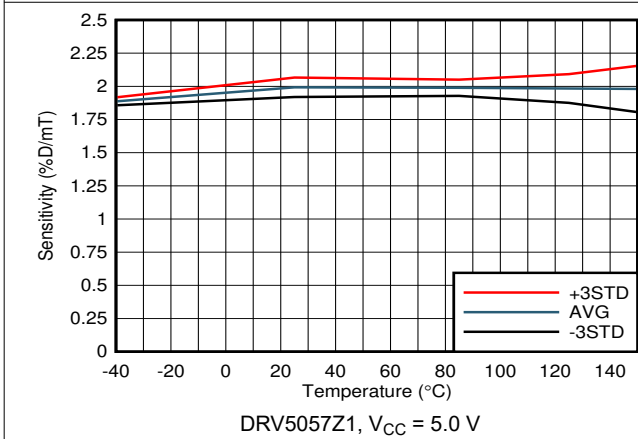
图 6-9. Sensitivity vs Temperature
