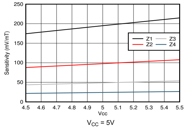
图 5-16. 灵敏度与电源电压之间的关系
