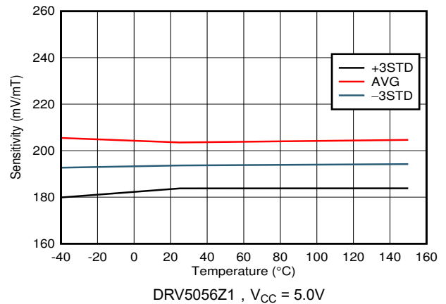
图 5-18. 灵敏度与温度之间的关系
