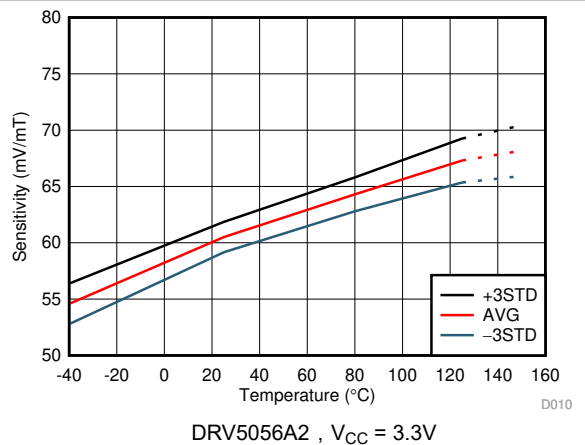
图 5-8. 灵敏度与温度之间的关系
