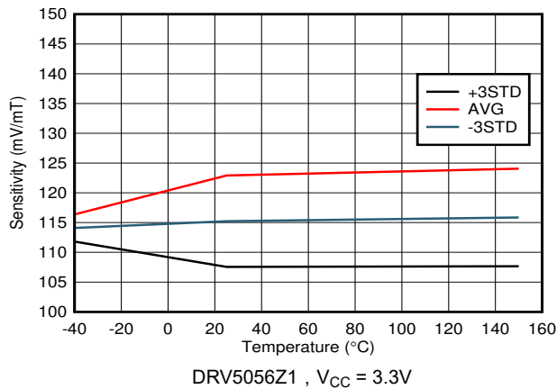
图 5-17. 灵敏度与温度之间的关系
