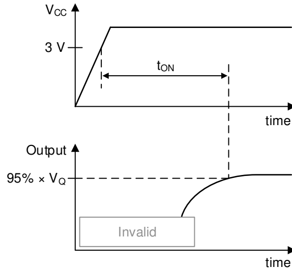
图 6-4. t_{ON} 定义
