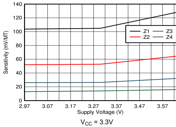
图 5-15. 灵敏度与电源电压之间的关系
