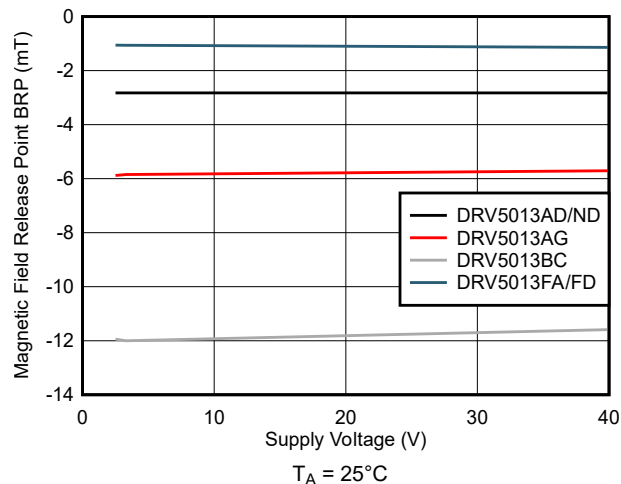
图 5-7. B_{RP} 与 V_{CC} 间的关系
