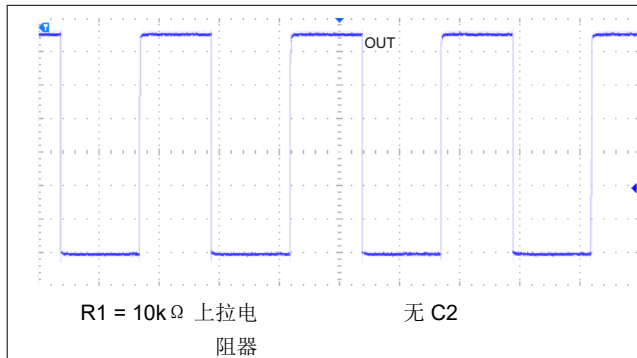
图 7-2. 10kHz 开关磁场
