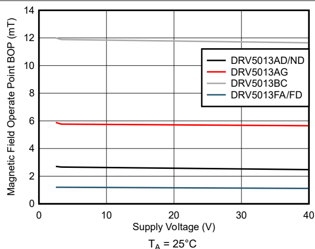
图 5-5. B_{OP} 与 V_{CC} 间的关系
