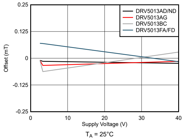
图 5-11. 偏移与 V_{CC} 间的关系
