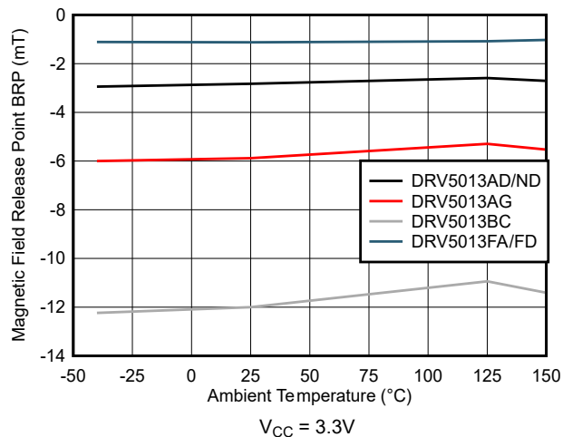
图 5-8. B_{RP} 与温度间的关系
