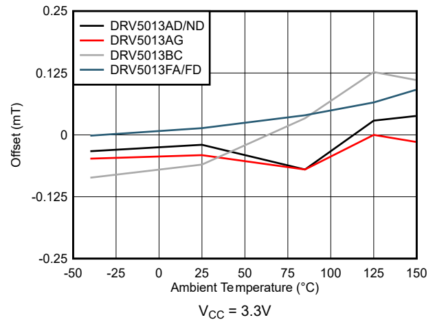
图 5-12. 偏移与温度间的关系
