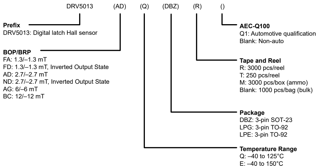
图 8-1. 器件命名规则
