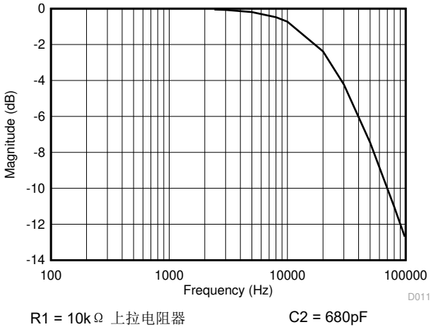
图 7-4. 低通滤波
