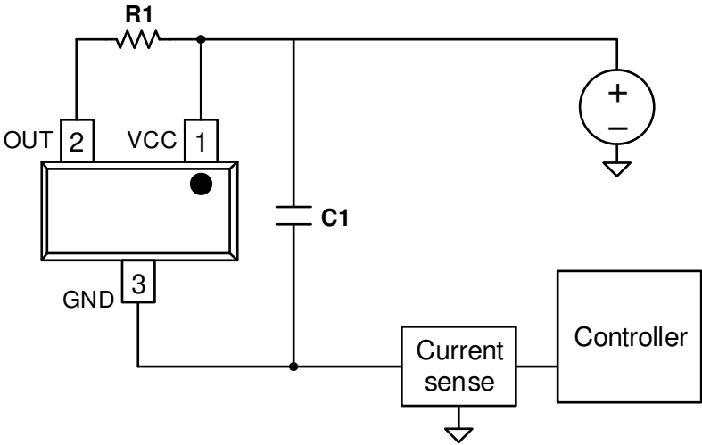
图 7-5. 两线制应用
