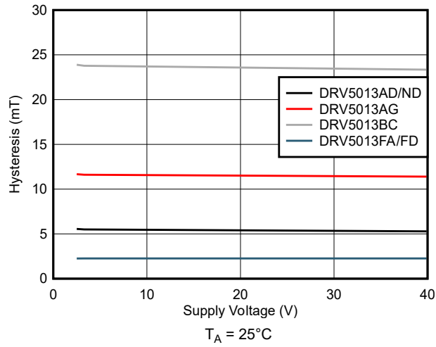
图 5-9. 迟滞与 V_{CC} 间的关系
