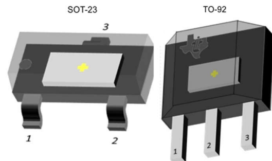
器件封装
