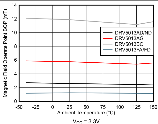
图 5-6. B_{OP} 与温度间的关系
