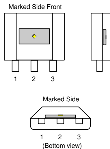
图 8-3. TO-92 (LPG、LPE) 封装
