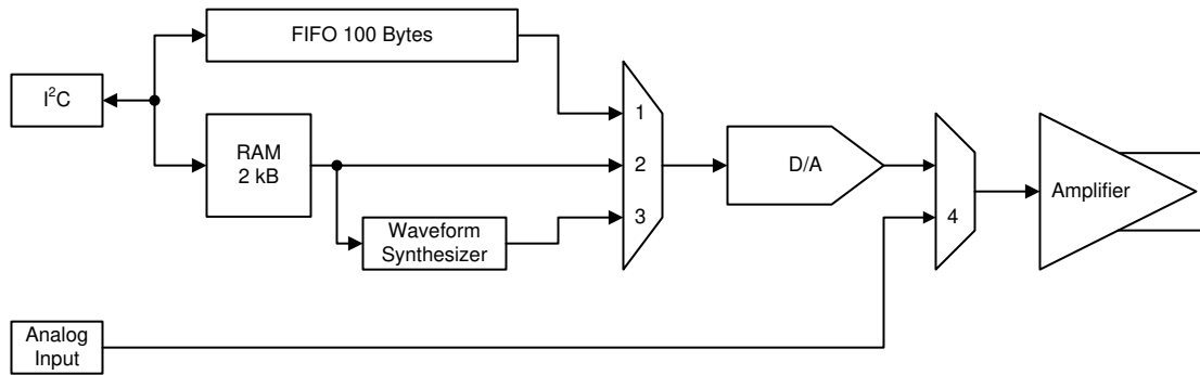
图 7-1. Front-End Interface
