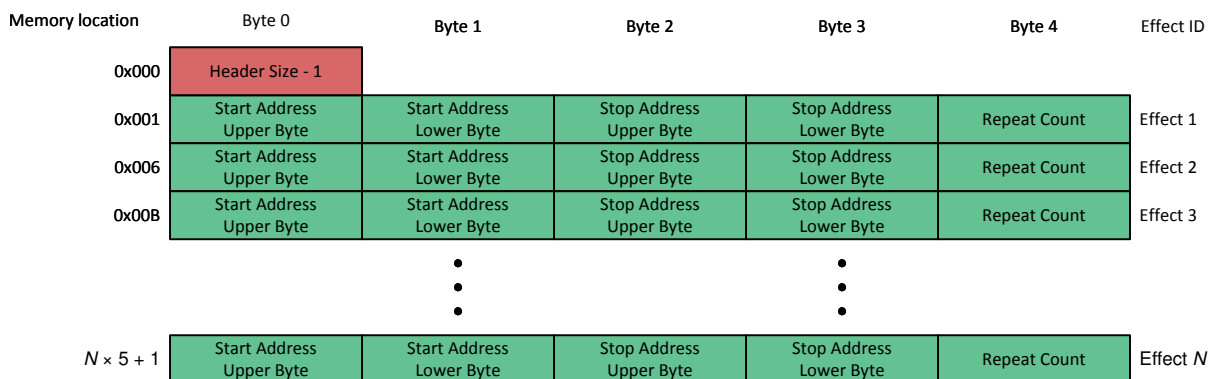
图 7-6. Header Format
