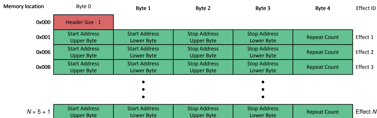
图 7-6. Header Format
