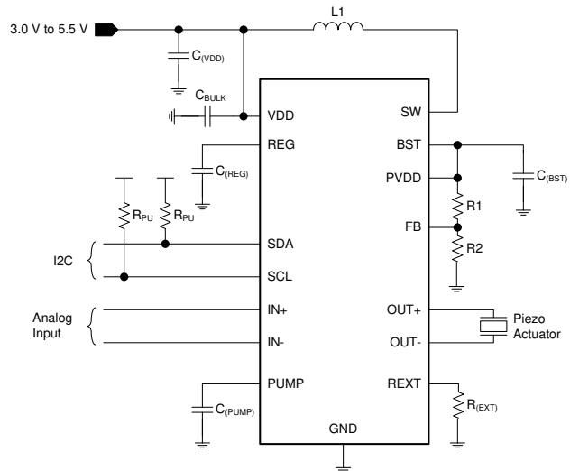
简化原理图
