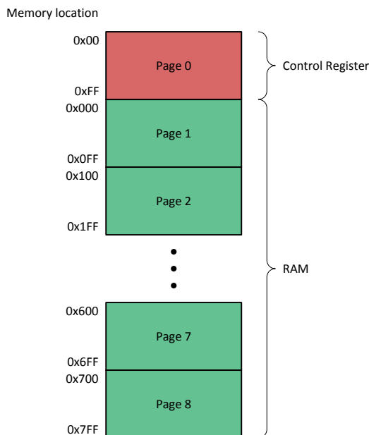
图 7-4. Page Structure
