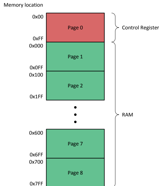
图 7-4. Page Structure
