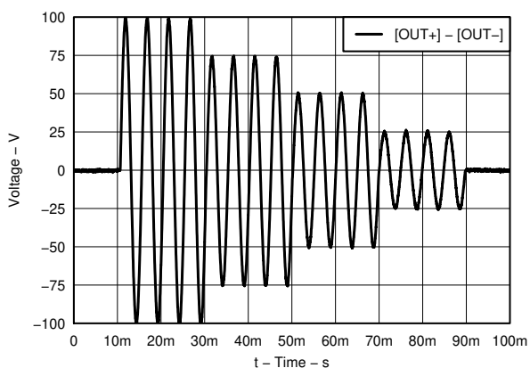
图 6-16. Example Waveform - Amplitude
