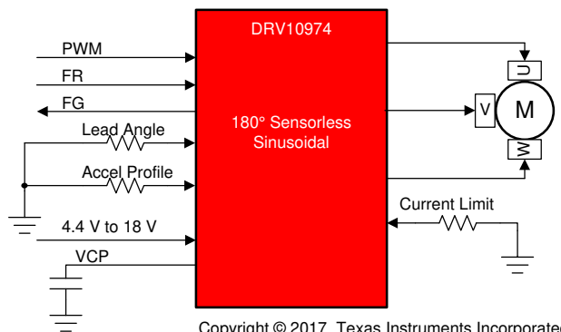
应用原理图
