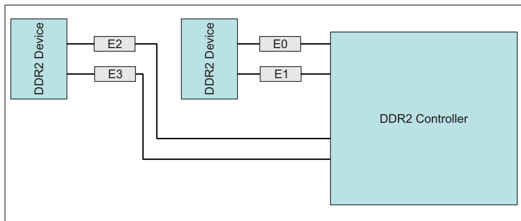
图 8-56. DQS and DQ Routing and Topology
