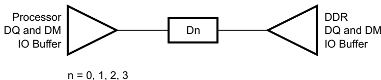
图 7-59. DQ/DM Topology
