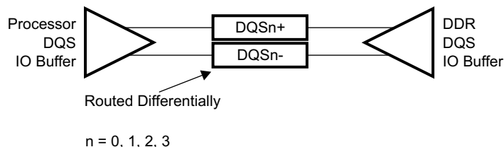
图 7-58. DQS Topology
