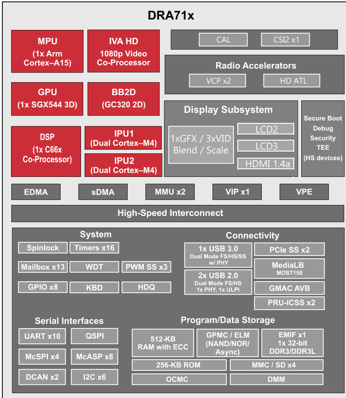
图 1-1. DRA71x 方框图
