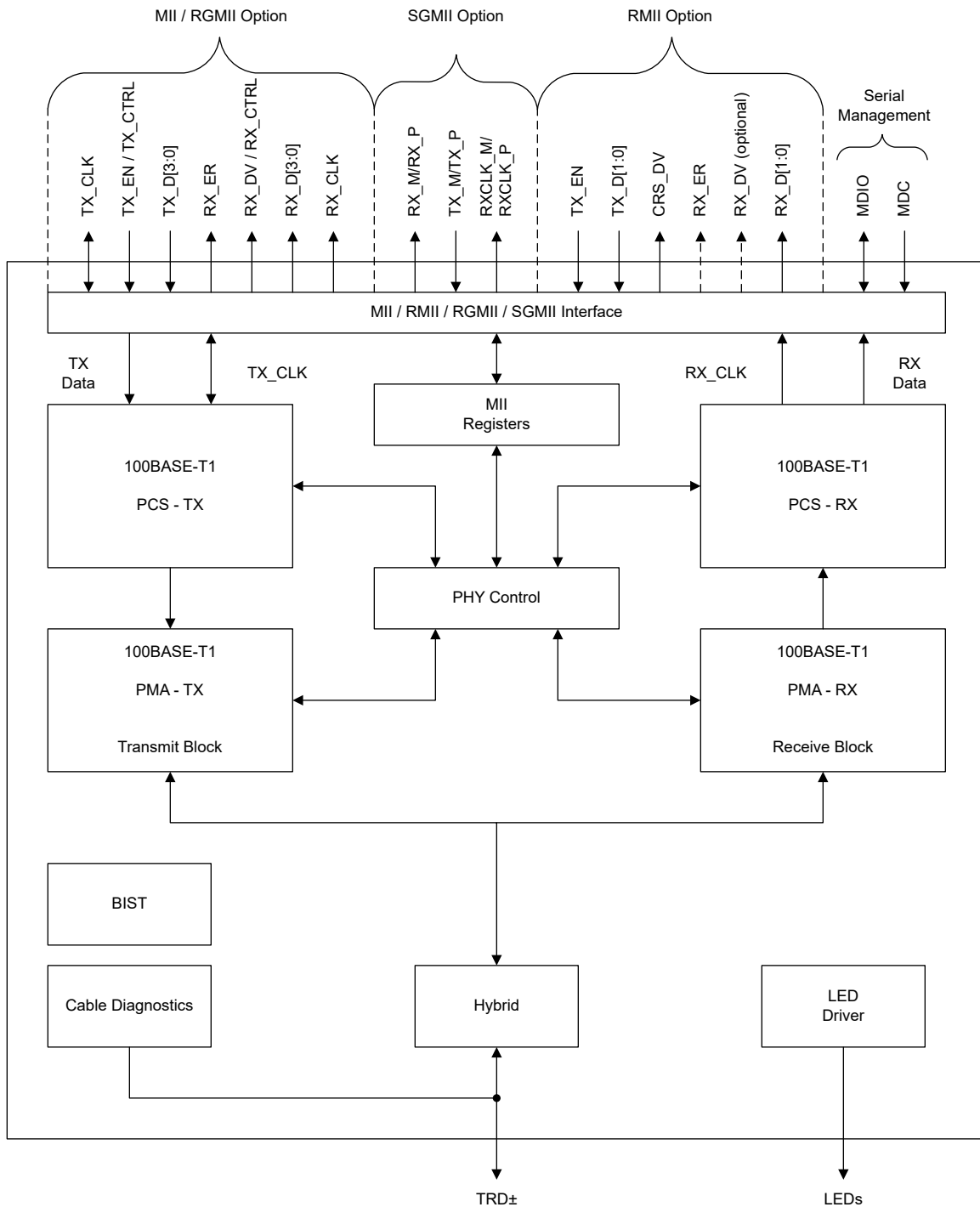
图 8-1. DP83TC814S-Q1
