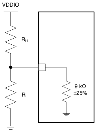
图 7-14. Strap Circuit
