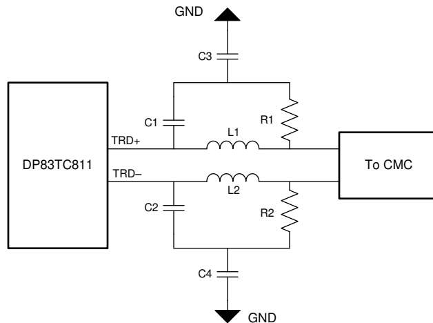
图 8-6. MDI Low-Pass Filter 1 2
