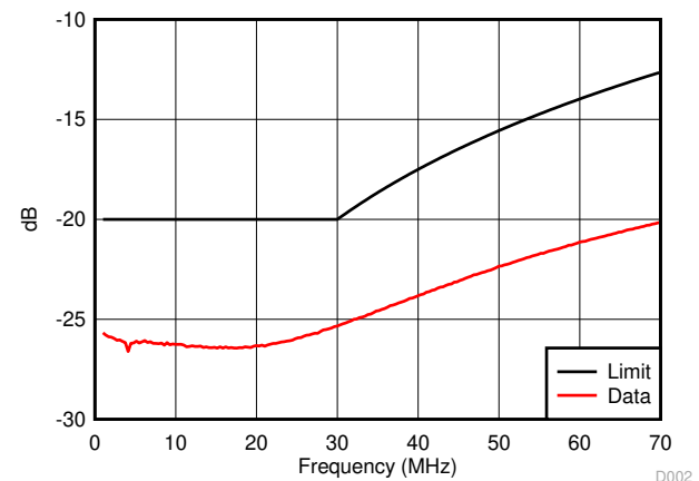
图 8-10. MDI Return Loss
